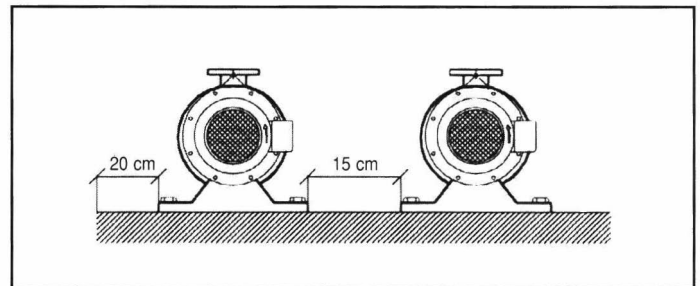
Şekil 21.22. İKİ POMPA ARASINDAKİ MESAFE
