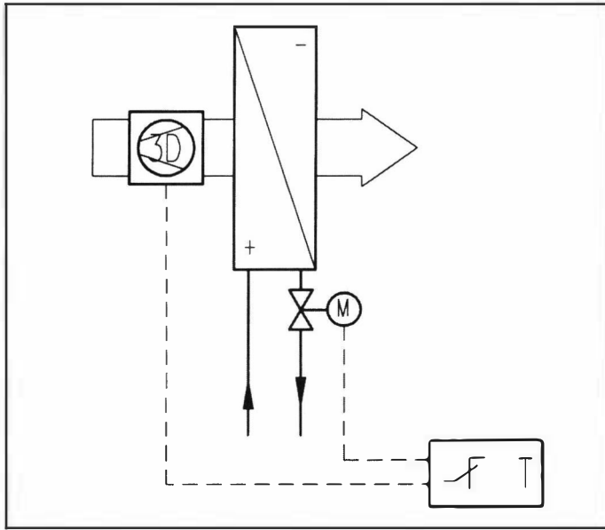
Şekil 11.15. İKİ YOLLU VANAYA KUMANDA.
