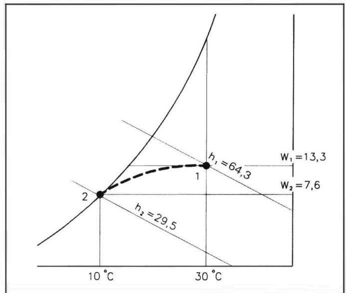
Şekil 10.9. ÖRNEK 3'ÜN PSİKROMETRİK DİYAGRAM YARDIMI İLE ÇÖZÜMÜ
