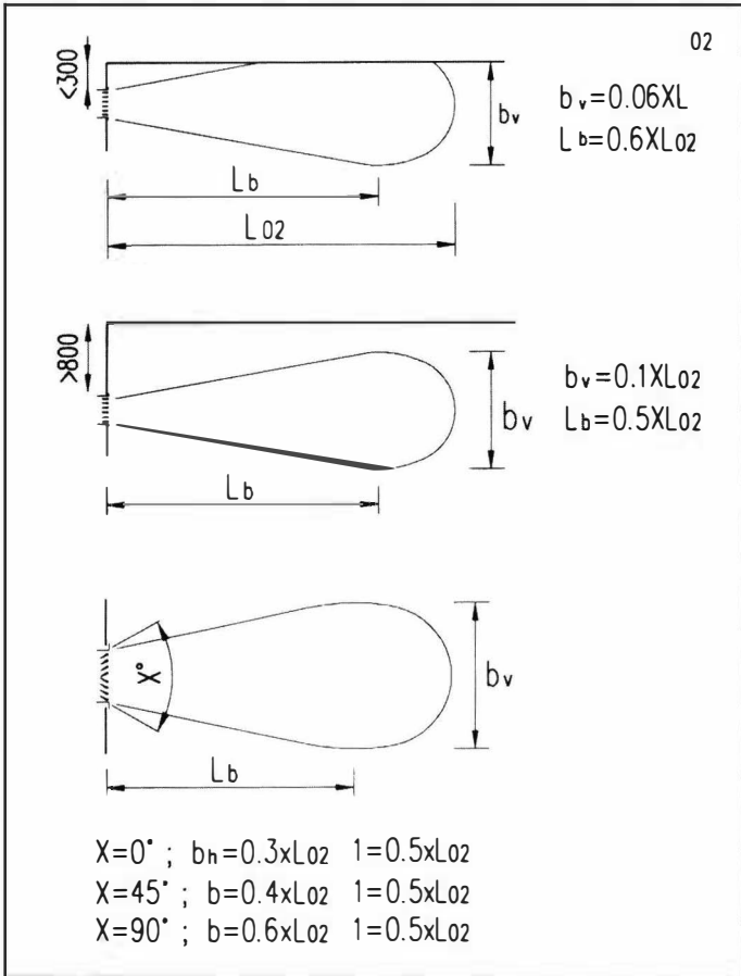
Şekil 4.24. JET ŞEKİLLERİ
