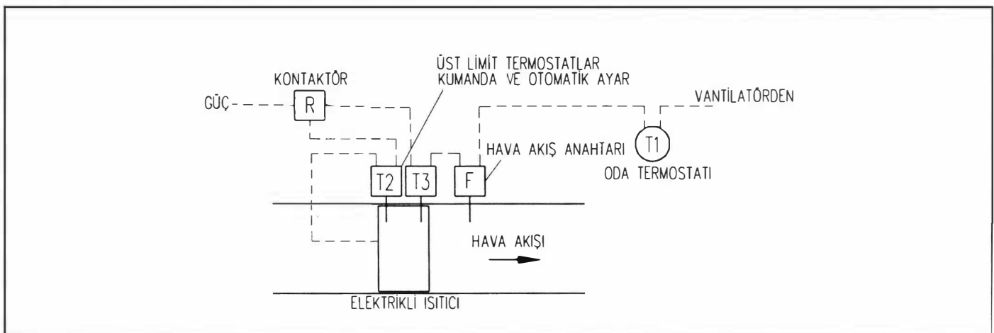
Şekil 18.21. KÜÇÜK KAPASİTELİ ISITICILARIN İKİ KONUMLU KONTROLÜ
