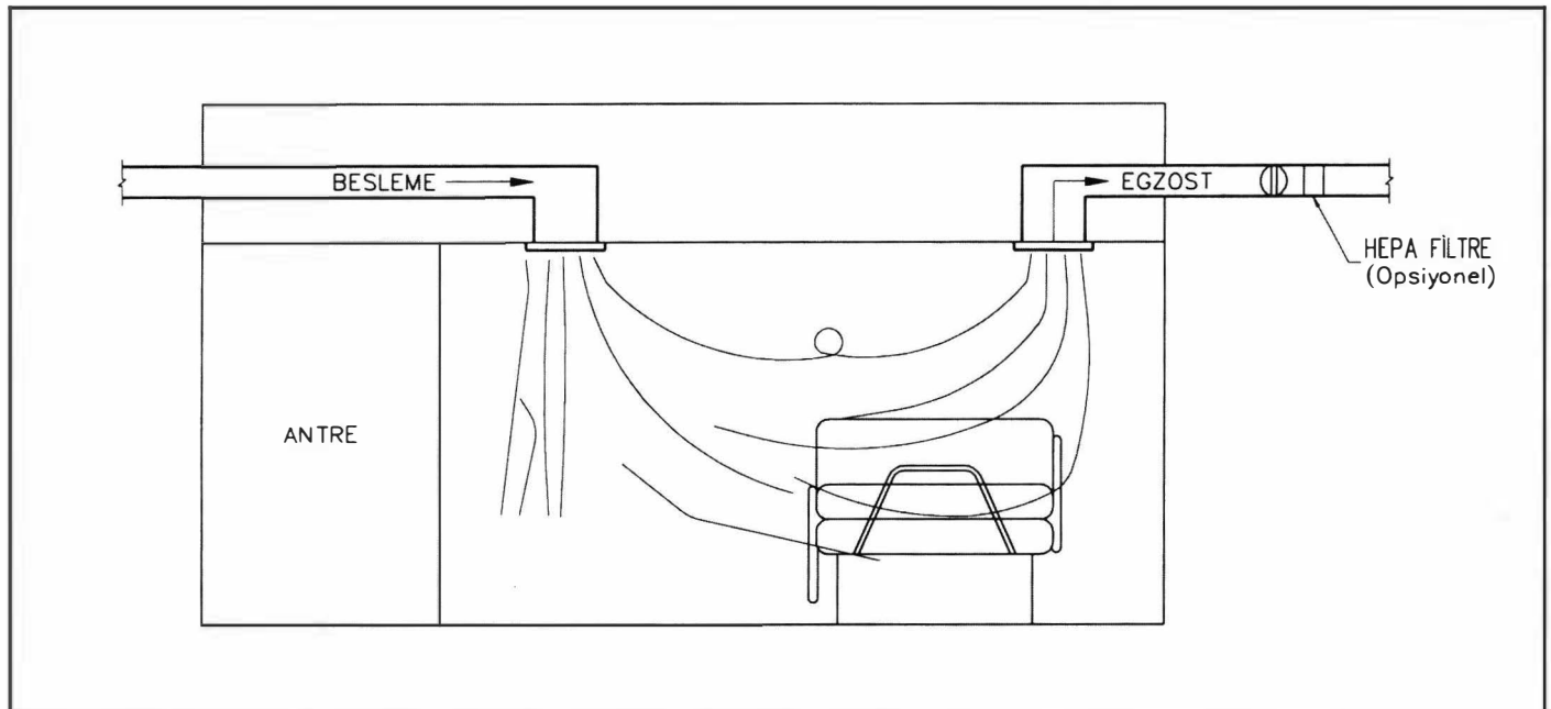
Şekil 16.10. TUM EGZOSU ATMOSFERE ATAN KARANTİNE ODASI HAVA AKIŞ BIÇIMI
