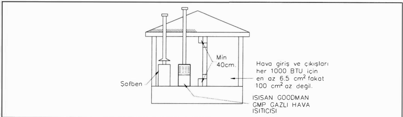
Şekil 12.52.B. İSİTİLAN HACİMİNDEN HAVA ALIMI
