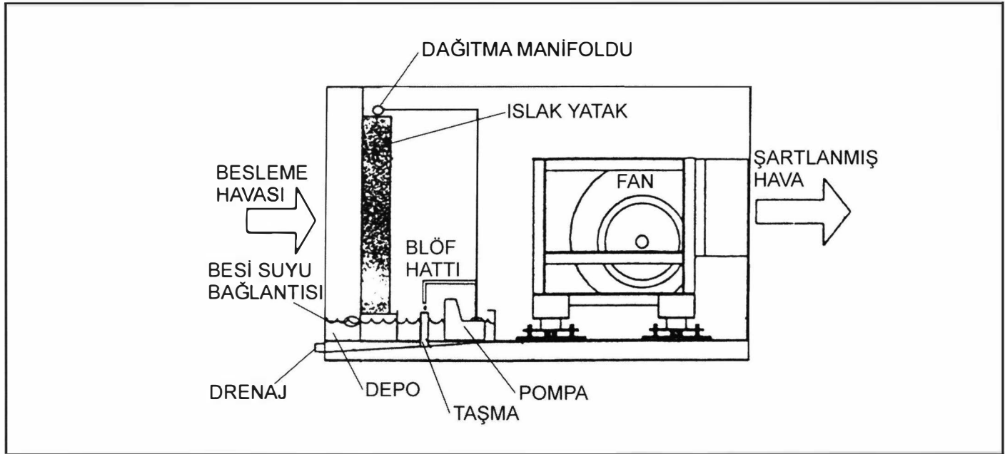
Şekil 5.7. EVAPORATİF SOĞUTUCULAR
