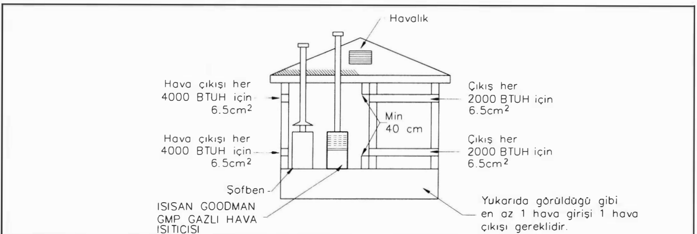
Şekil 12.52.C. YATAY GİRİŞ VE ÇIKIŞ KULLANILARAK DIŞ HAVA ALIMI
