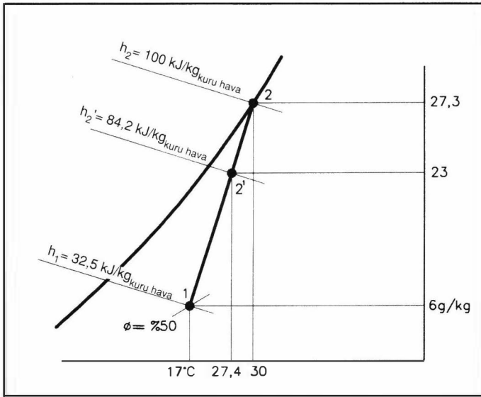
Şekil 10.19. ÖRNEK 10'UN PSİKROMETRİK DİYAGRAMDA ÇÖZÜMÜ
