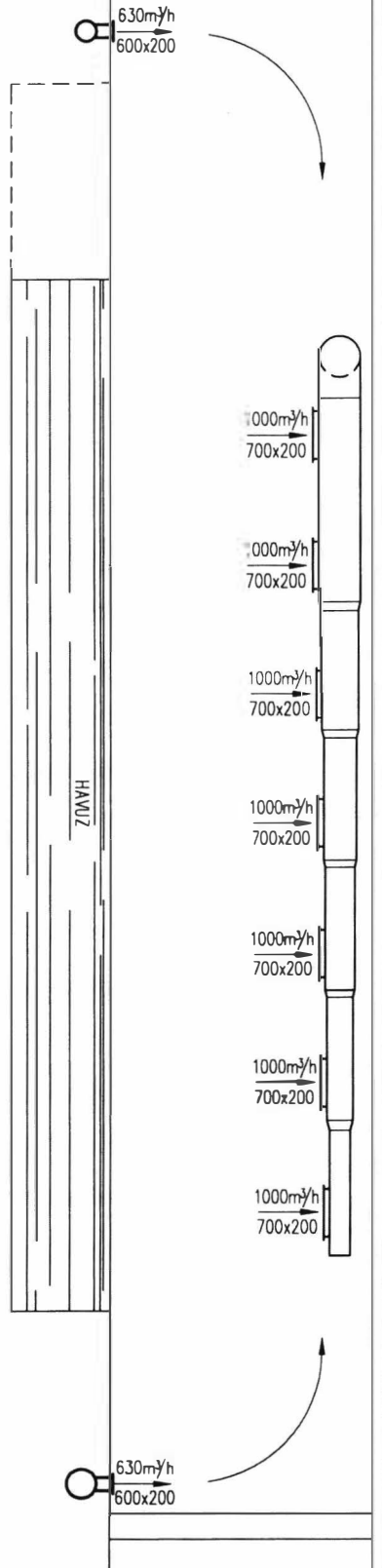
Şekil 14.36.B. ÖRNEK PROJE KESİT RESİMLERİ
