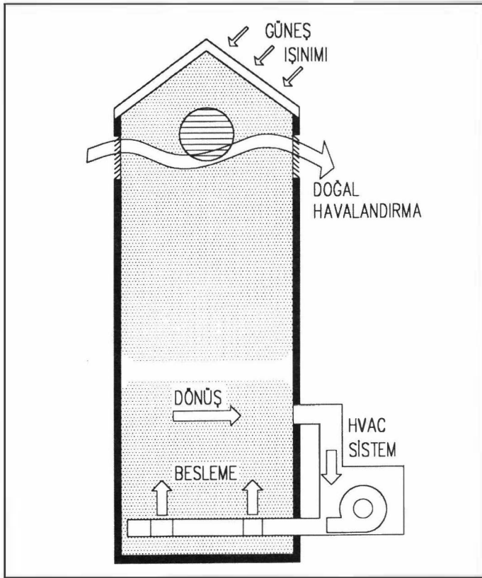
Şekil 14.19. YAZ ÇALIŞMASI HAVALANDIRMASI
