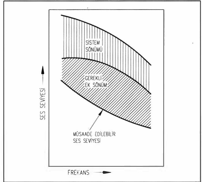
Şekil 2.5. EK SÖNÜMLEYİCİ SEÇİMİNİN PRENSİBİ
