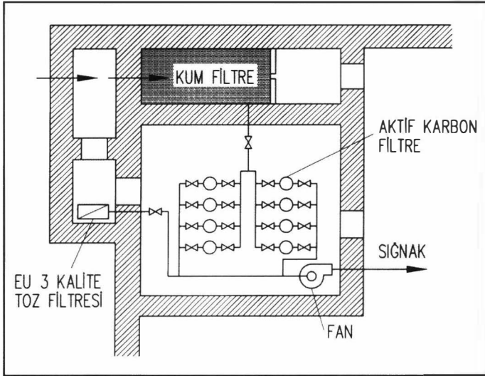
Şekil 14.47. SİĞINAK HAVALANDIRMA TESİSAT ŞEMASI
