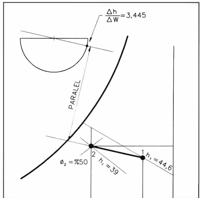
Şekil 10.23. ÖRNEK 12'NİN PSİKROMETRİK DİYAGRAMINDA GÖSTERİMİ
