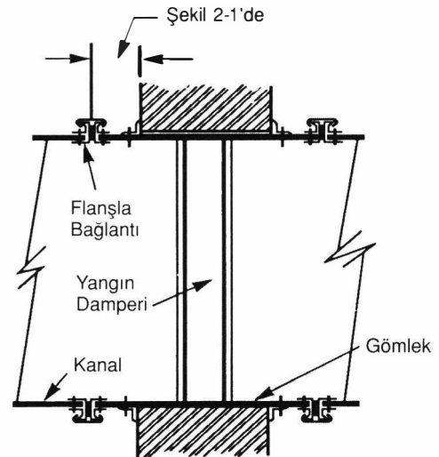
Şekil 6.19. UL TESTİNDEN GEÇMİŞ DAMPER BAĞLANTILARI
