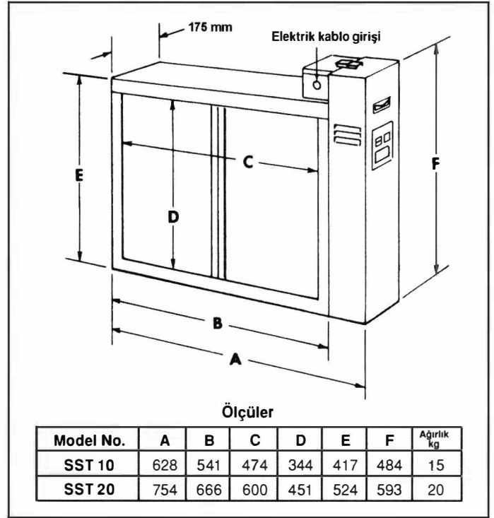
Şekil 12.78. ELEKTROSTATİK FİLTRE
