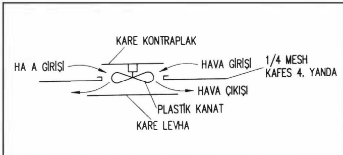
Şekil 14.64. BESLEME FANI DETAYI
