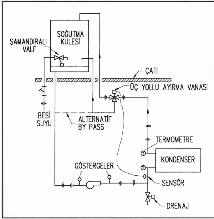
Şekil 17.19. BY-PASS HATLI KULE DEVRESİ
