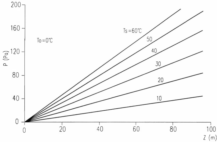
Şekil 6.11. BACA ETKİSİNİN YÜKSEKLİK VE SICAKLIKLA DEĞİŞİMİ
