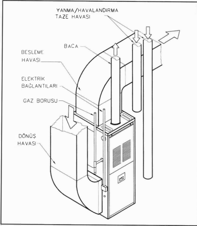
Şekil 12.47. ISISAN GOODMAN GMP HAVA ISITICISI DİKEY MONTAJ
