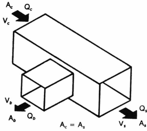
EK 2. Şekil 20. T PARÇA, BRANŞMAN VE ANA KANAL DİKDÖRTGEN
