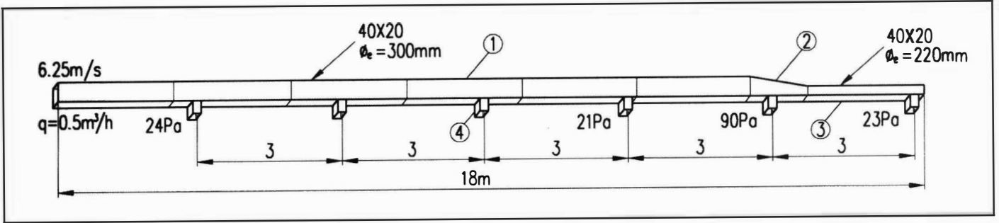
Şekil 1.74. SİSTEM A, DİKDÖRTGEN
