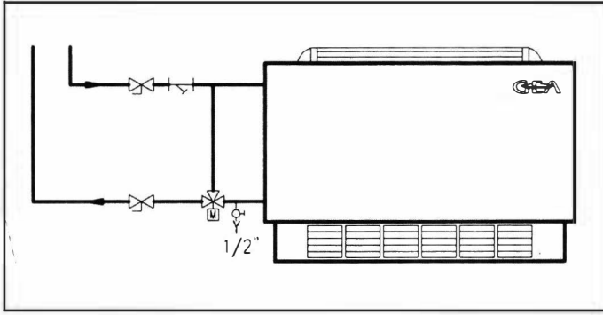
Şekil 21.18. BOŞALTIMA MUSLUĞU
