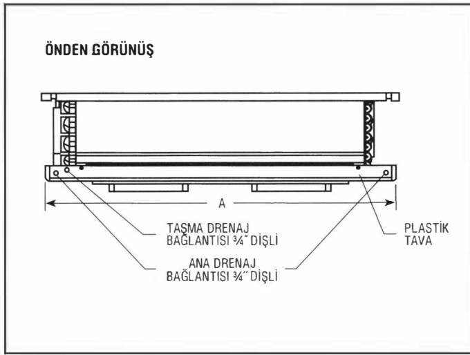
Şekil 12.29. GİZLİ TAVAN TİPİ KANALLI KLİMA
