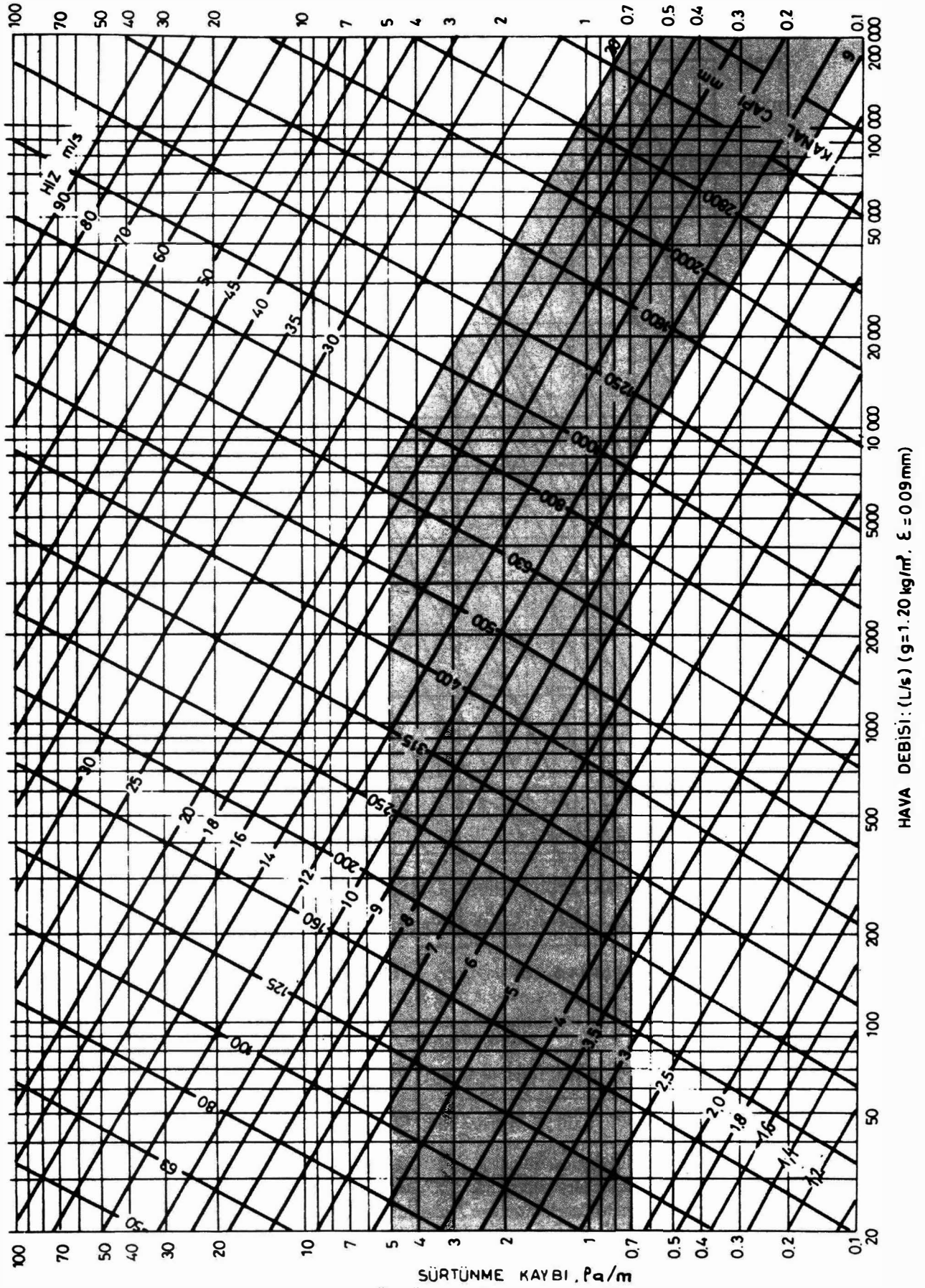
Şekil 1.22. SÜRTÜNME DİYAGRAMI
