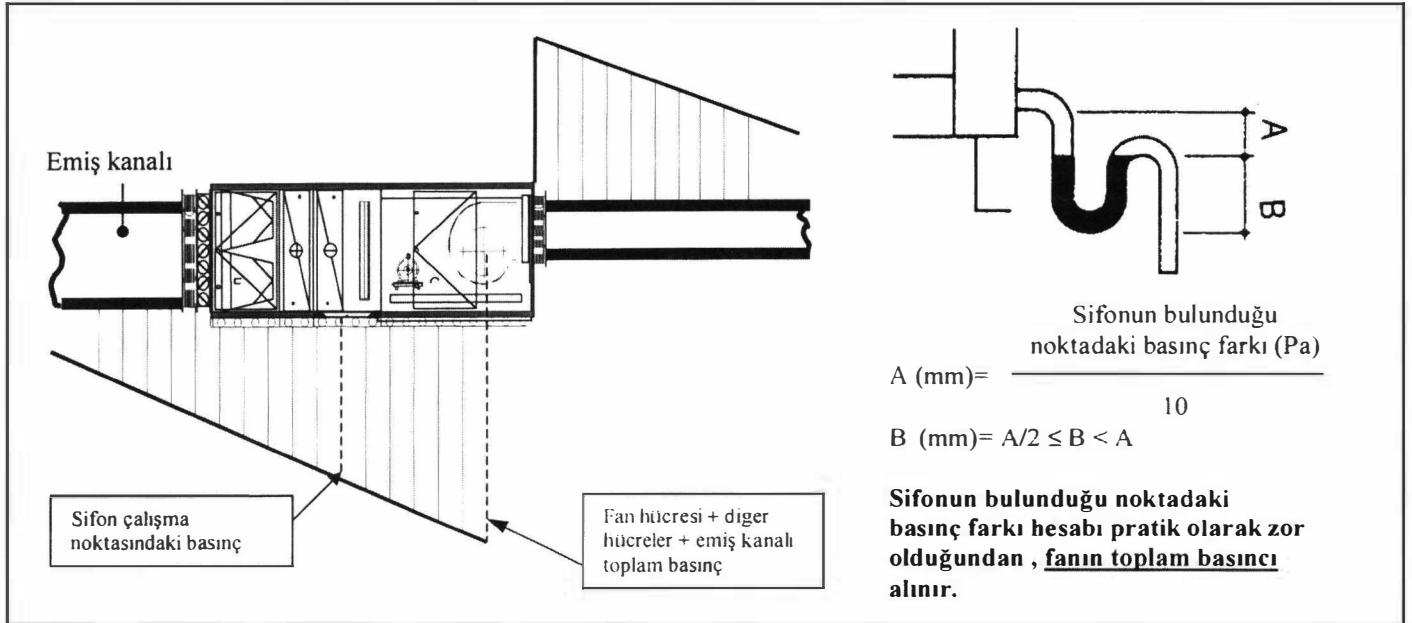
Şekil 17.49. SİFON HESABI
