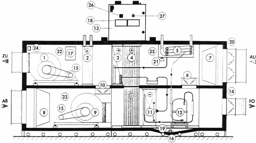
Şekil 14.41. ÖZEL HAVUZ KLİMA SANTRALI
