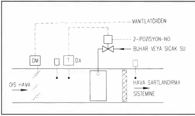
Şekil 18.10. ÖN ISITMA KONTROLÜ
