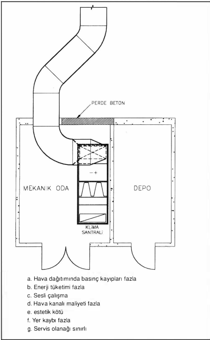
Şekil 1.62. ANA KANAL DÜZENLEMESİNDE YANLIŞ ÇÖZÜM
