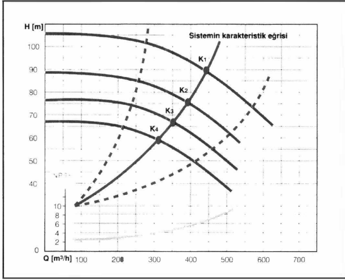
Şekil 17.106. POMPA VE SİSTEMİN KARAKTERİSTİK EĞRİLERİ
