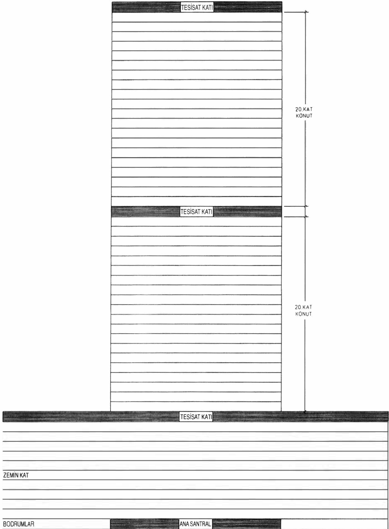
Şekil 15.1. İÇ ZON VAV, ÇEVRE ZONU VAV + RADYATÖRLE STATİK ISITMA SİSTEMİ
