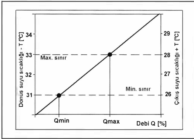
Şekil 17.116. GİDİŞ VEYA DÖNÜŞ SUYU SICAKLIK KONTROLÜ
