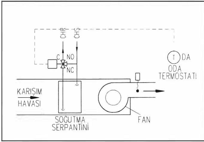
Şekil 18.16. ÜÇ YOLLU VANA İLE KONTROL
