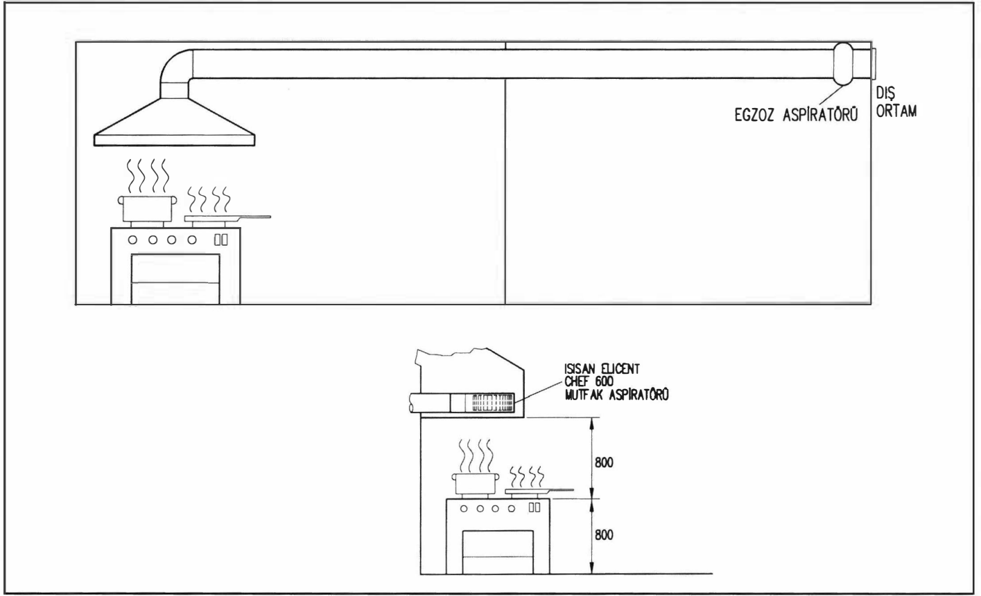
Şekil 14.5. MUTFAK ASPIRATÖRÜNÜN KANALLA YANDAN DIŞARI BAĞLANMASI
