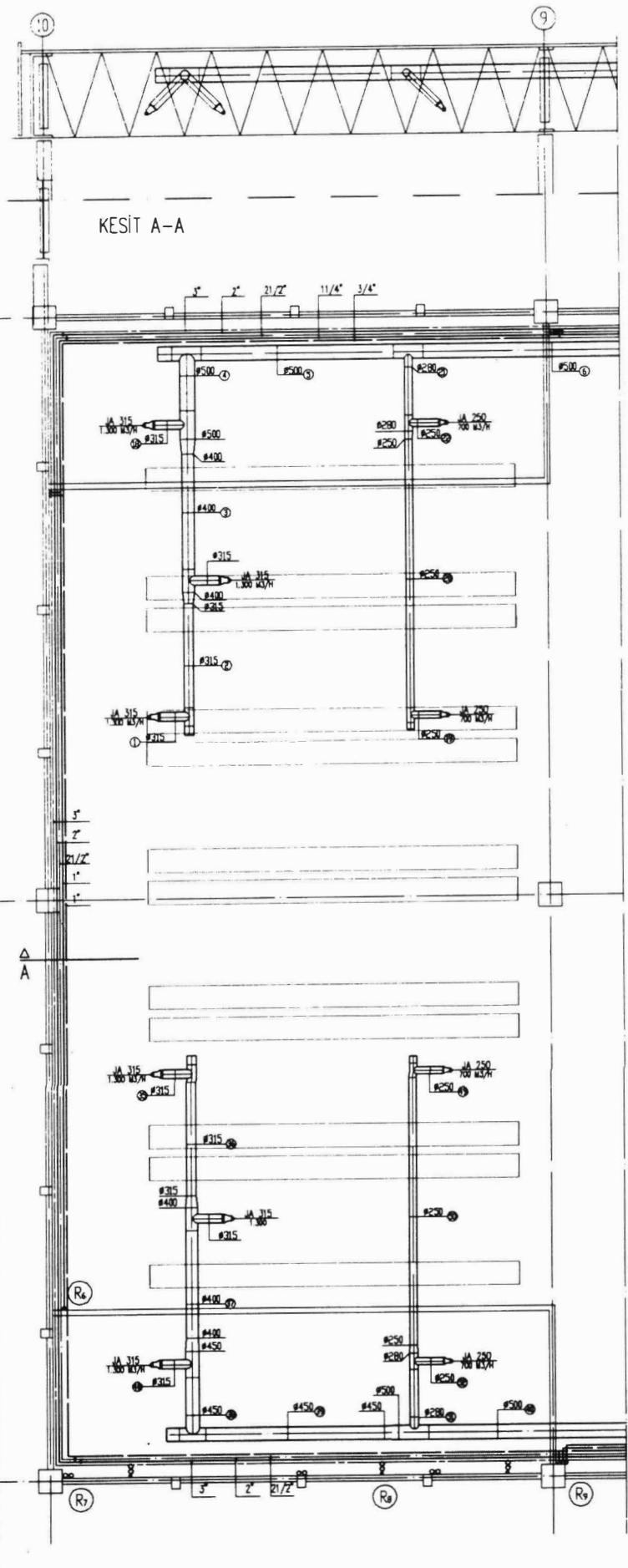
Şekil 14.67.A. BOYA ATÖLYESİ HAVALANDIRMA PROJESİ
