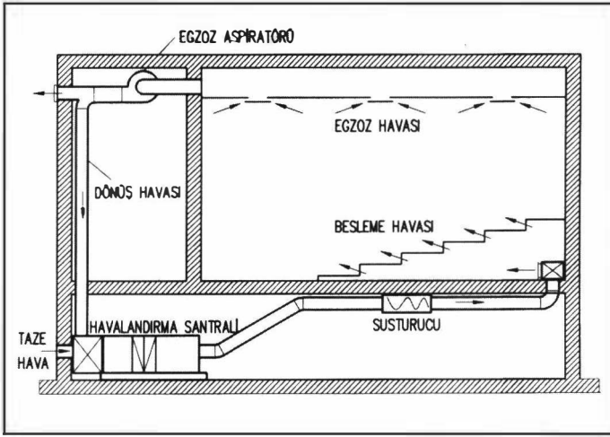
Şekil 14.28. AŞAĞIDAN YUKARI DOĞRU HAVALANDIRMA
