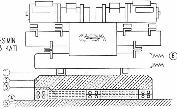
Şekil 17.6. KAİDE DETAYI
