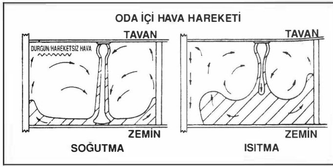
Şekil 4.17. GRUP E ÇIKIŞLARI HAVA HAREKETİ KARAKTERİSTİKLERİ
