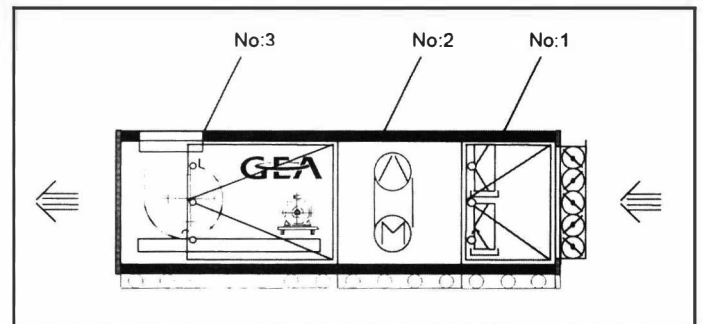
Şekil 17.60. TEK FİLTRASYON KADEMELİ MUTFAK ASPİRATÖRÜ
