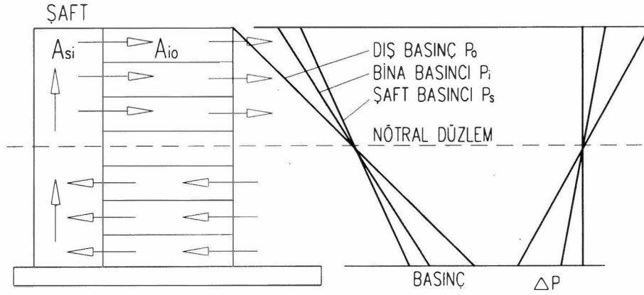
Şekil 6.10. NORMAL BACA ETKİSİ DURUMUNDA OLUŞAN BASINÇ DAĞILIMI
