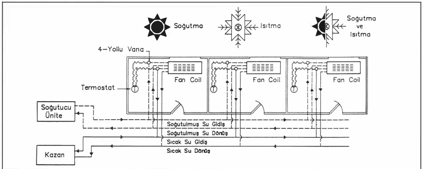
Şekil 11.11. 4 BORULU SİSTEM
