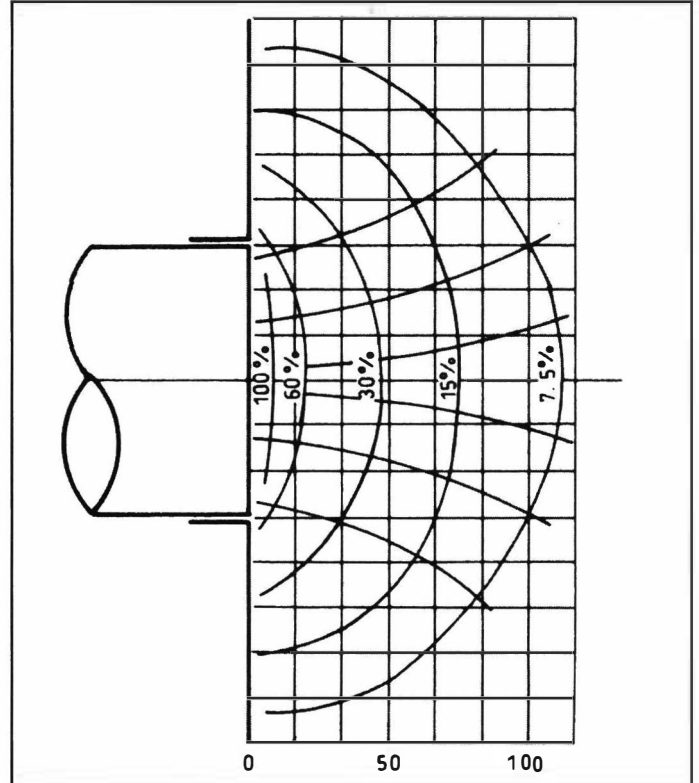
Şekil 7.14. HIZ KONTURLARI - FLANŞLI DAİRESEL AÇIKLIKLAR - AÇIKLIK HIZININ %'Sİ
