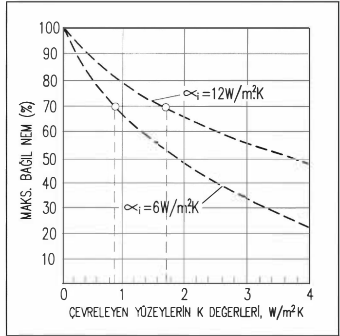
Şekil 14.37. YÜZEYLERDE YOĞUŞMA KOŞULLARI
