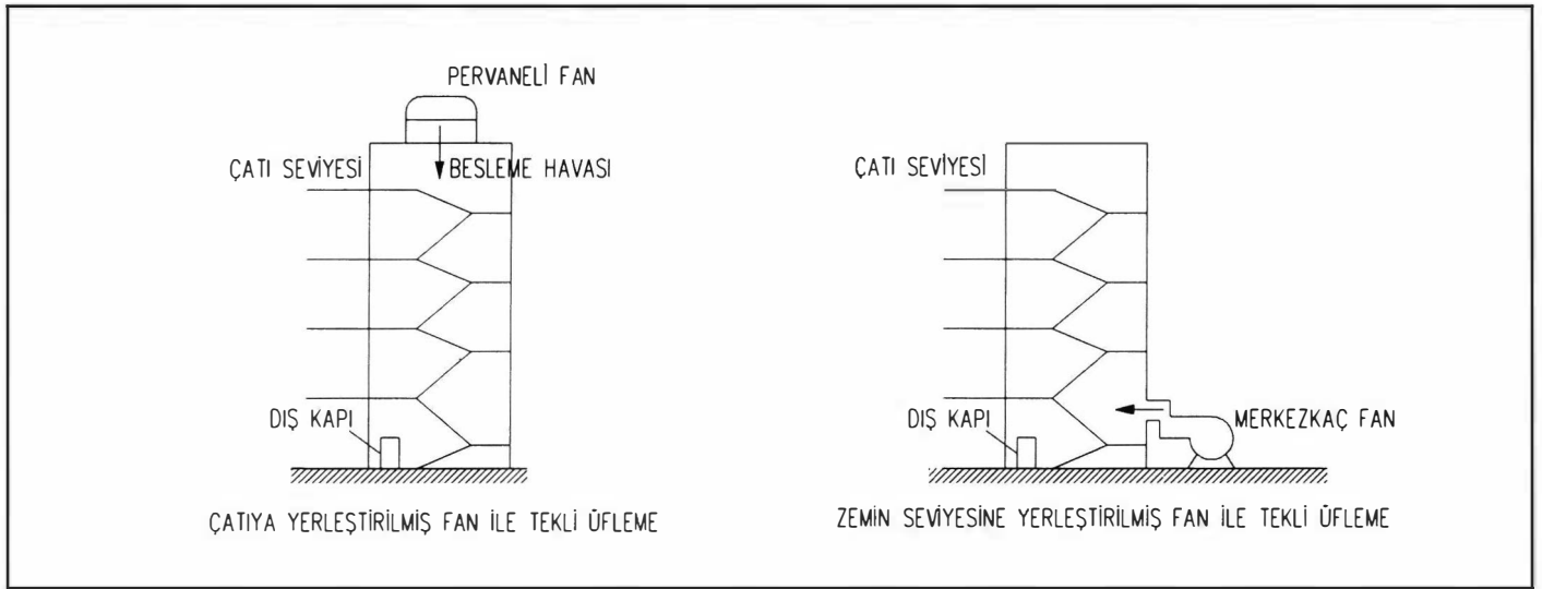
Şekil 6.12. MERDİVEN YUVASININ ALT VE ÜST KISIMLARINDA TEK Lİ ÜFLEME
