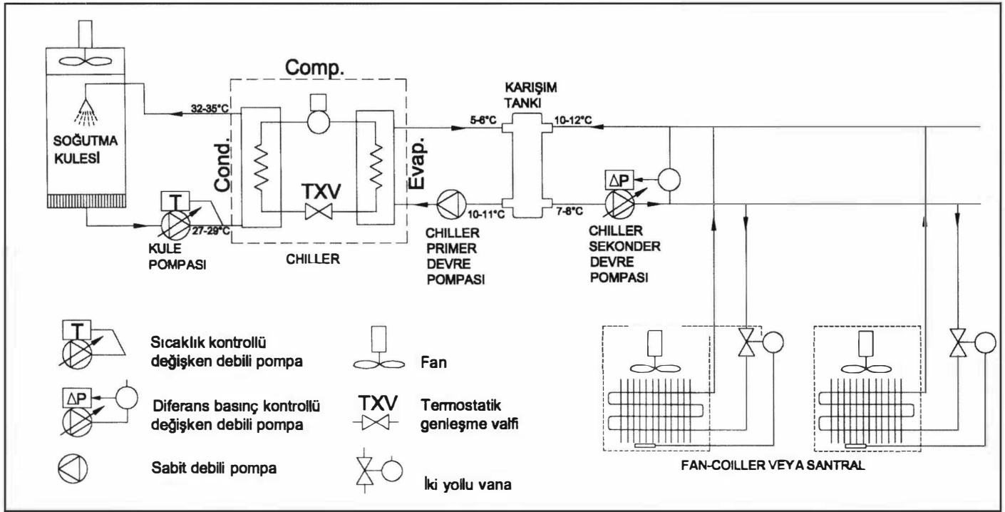
Şekil 17.98. BİR SOĞUTMA DEVRESİNDE KULLANILAN SİRKÜLASYON POMPALARININ UYGULAMA ÖRNEĞİ
