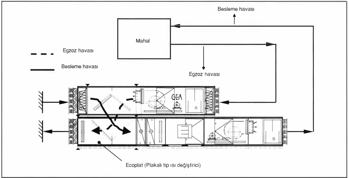
Şekil 17.52. PLAKALI ISI DEĞİŞTİRİCİ KULLANAN ISI GERİ KAZANIMLI SANTRAL
