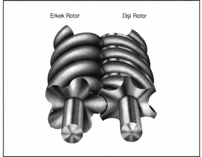
Şekil 17.11. ÇİFT VİDALI KOMPRESÖR
