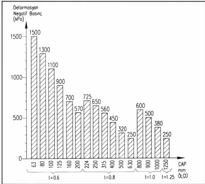
Şekil 1.68. SİRAL KANALLAR POZİTİF BASINÇ DAYANIMI
