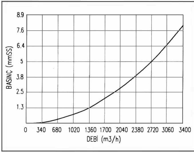
Şekil 1.47. SERPANTİNDEKİ BASINÇ DÜŞÜMÜ
