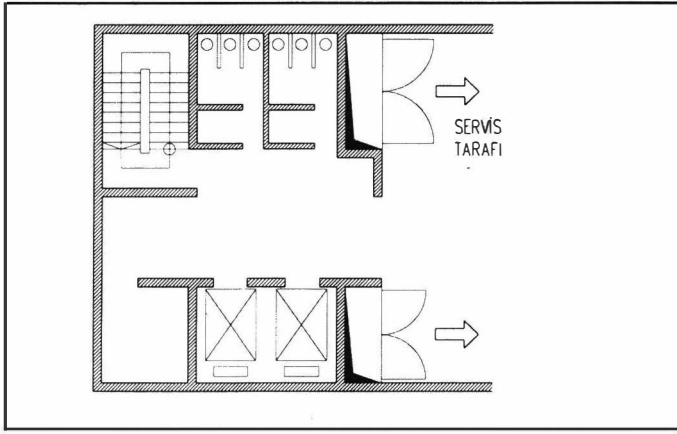
Şekil 1.57. 5 KATLI BİR İŞYERİ BİNASININ ÇEKİRDEĞİ
