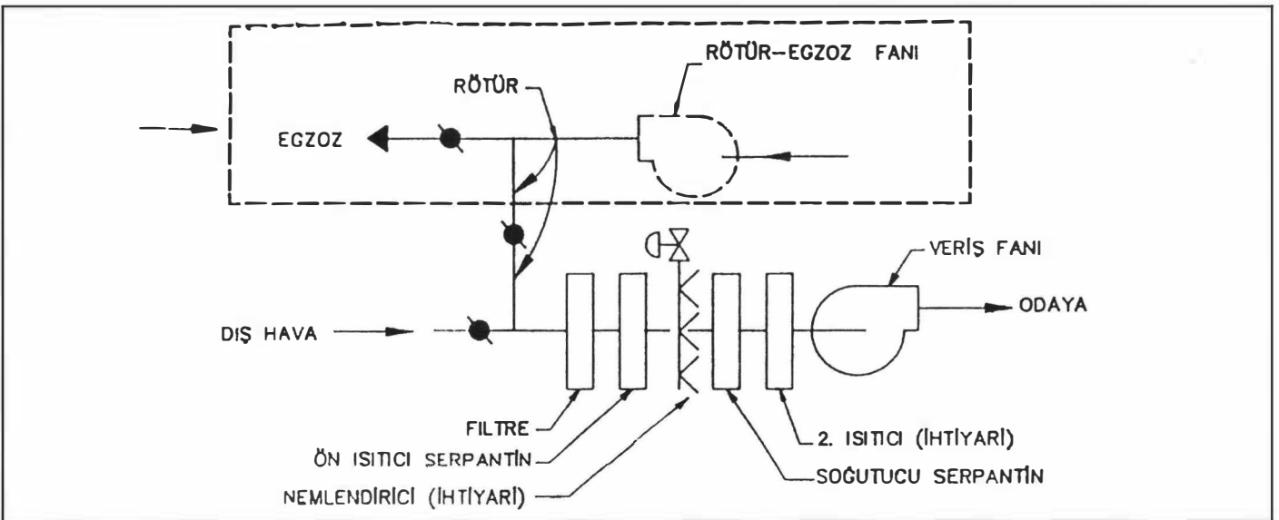
Şekil 11.1. TEK KANALLI SİSTEM
