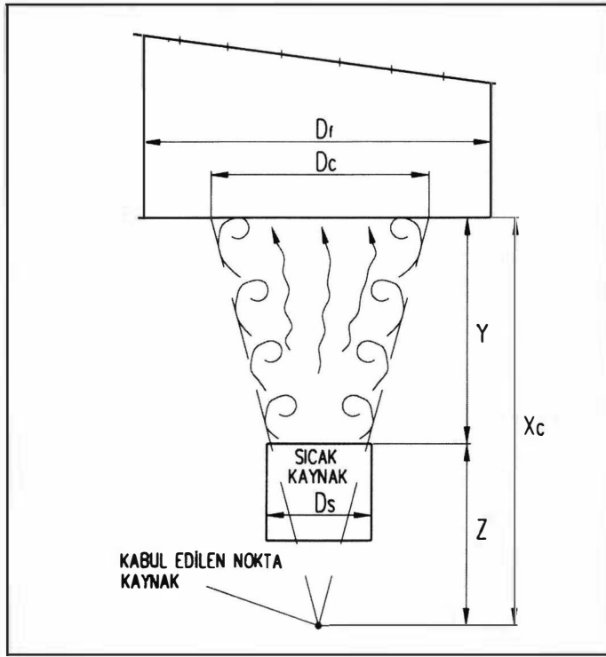
Şekil 7.16. SICAK KAYNAKLAR İÇİN YÜKSEK KANOPI DAVLUMBAZLARININ DİZAYNI İÇİN KULLANILAN BOYUTLAR
