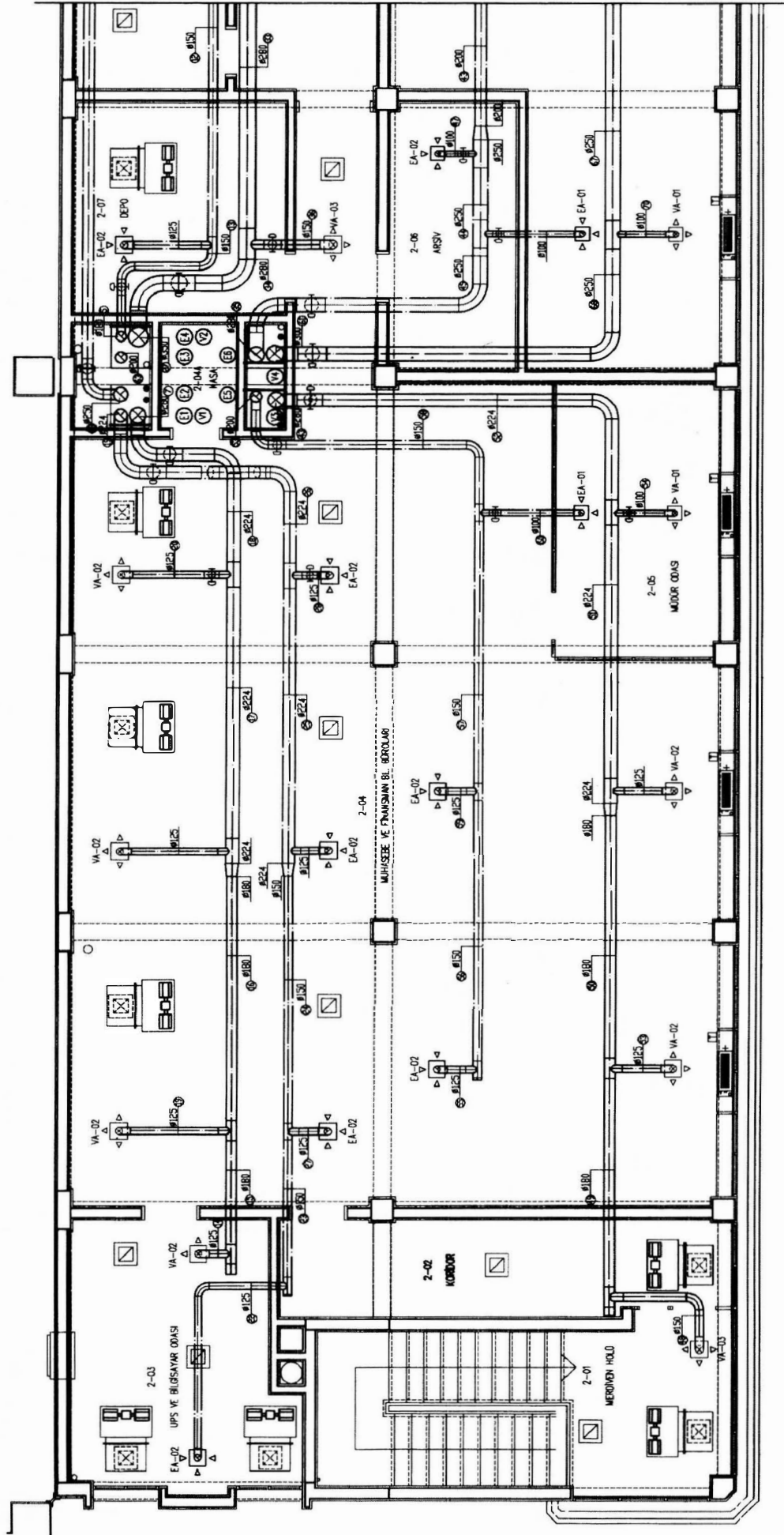
Şekil 14.10.B. ÖRNEK OFİS TAZE HAVA BESLEME SİSTEMİ PLAN GÖRÜNÜŞÜ
