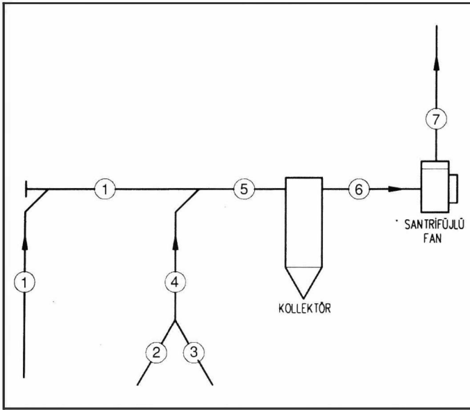
Şekil 1.35. BÖLÜM NUMARALARI İLE SİSTEM ŞEMASI
