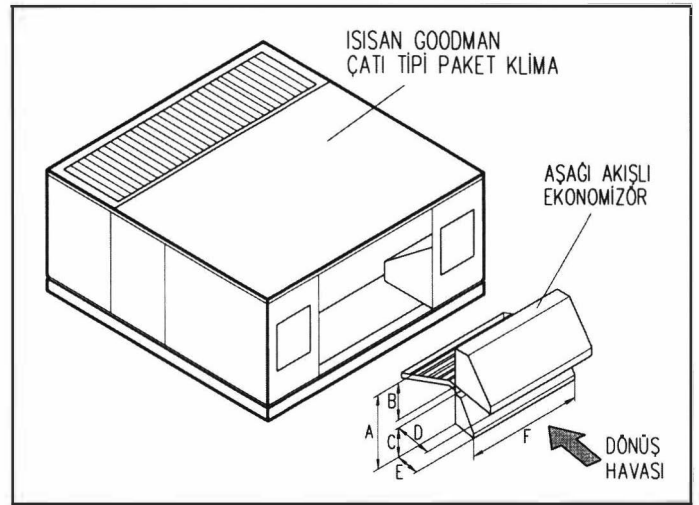
Şekil 12.71. AŞAĞI AKIŞLI EKONOMİZÖR
