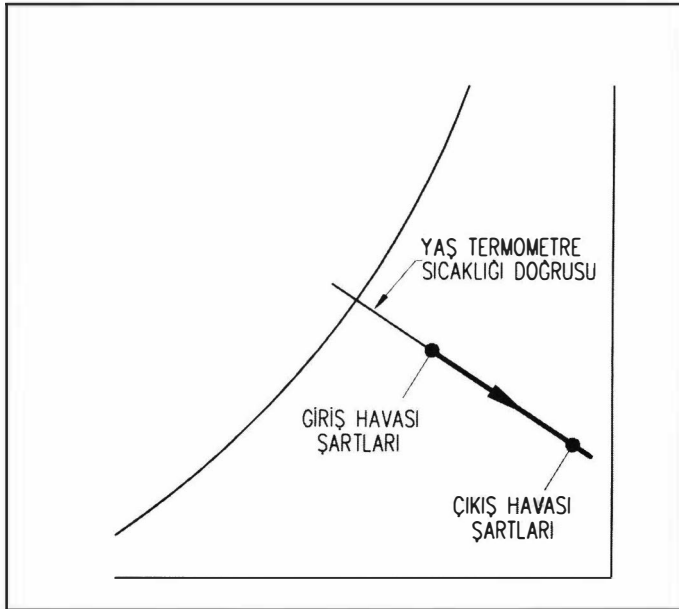
Şekil 10.20. NEM ALICI MADDELERLE HAVANIN NEMİNİN ALINMASI
