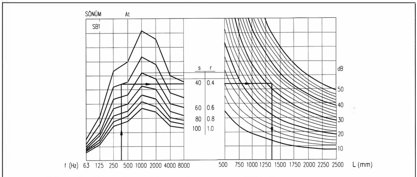
Şekil 2.23. SÖNÜM ABAĞI
