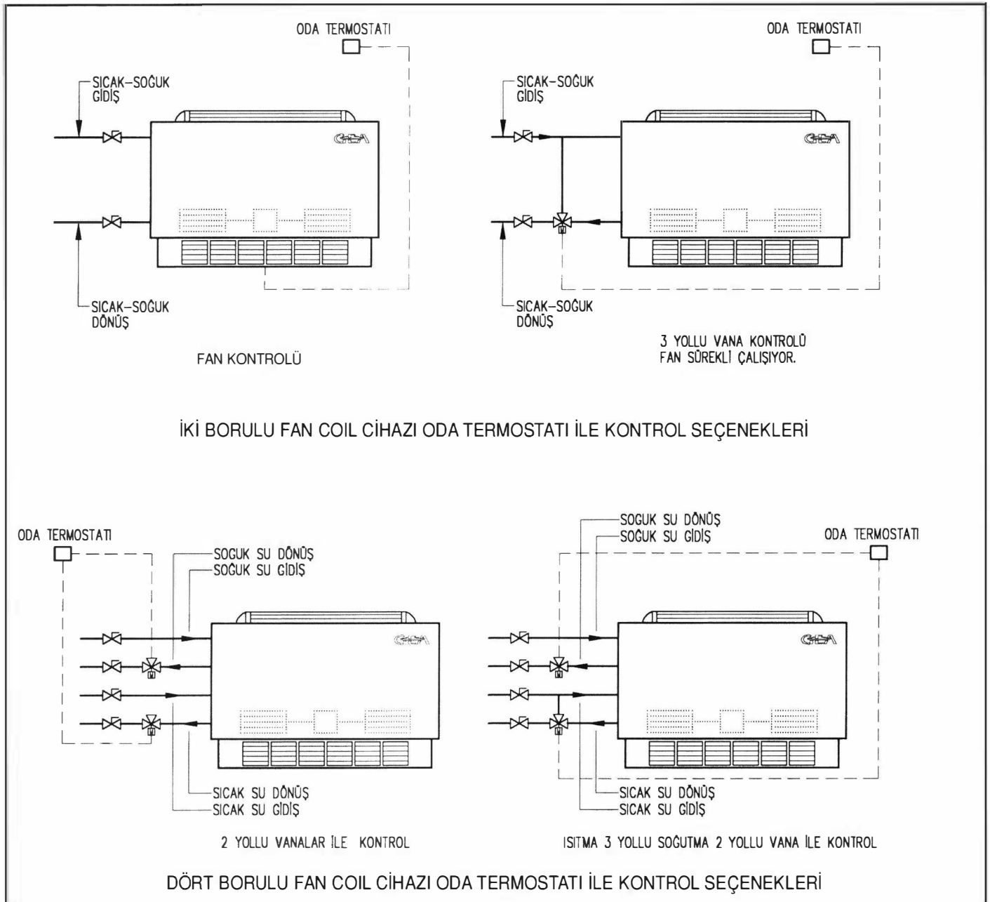
Şekil 17.79. FAN COIL OTOMATİK KONTROL ŞEKİLLERİ
