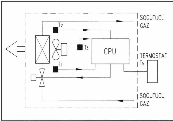
Şekil 11.20. DEĞİŞKEN SOĞUTUCU AKIŞKAN DEBİLİ SİSTEM İÇ ÜNİTESİ
