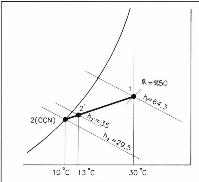
Şekil 10.10. ÖRNEK 4'ÜN PSİKROMETRİK DİYAGRAMINDA GÖSTERİMİ
