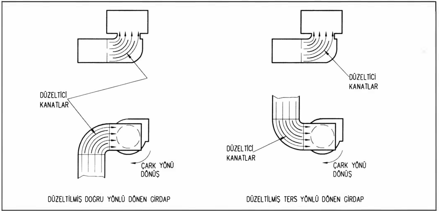
Şekil 1.30. GİRİŞ GİRDAPLARI İÇİN DÜZELTMELER
