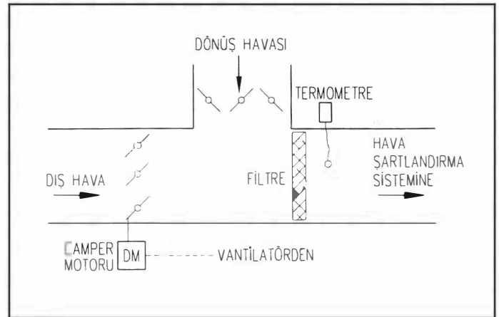
Şekil 18.6. MİNİMUM DİŞ HAVA KONTROLU
