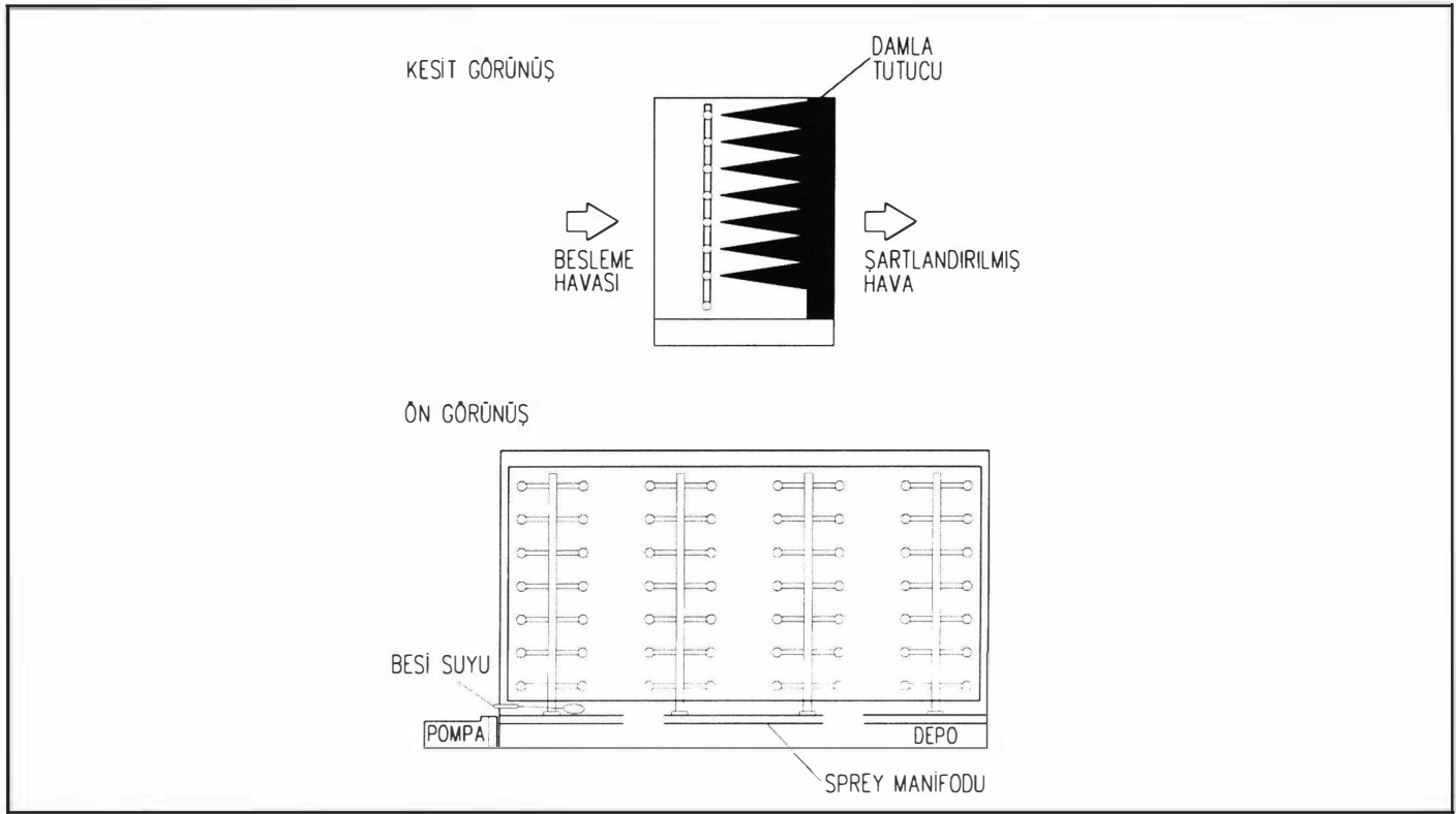
Şekil 5.8. YIKAMALI NEMLENDİRİCİ
