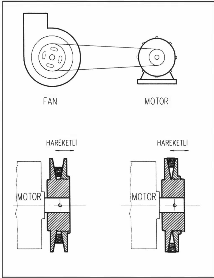
Şekil 12.63. KAYIŞ KASNAK MEKANİZMASI
