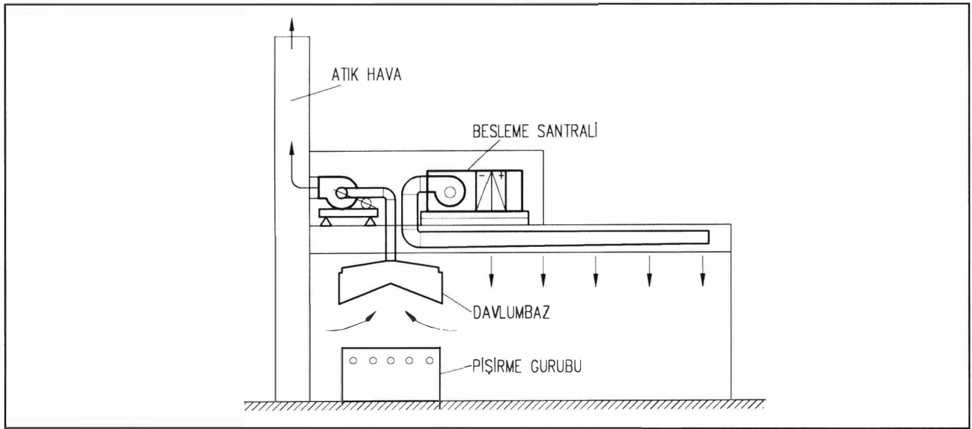
Şekil 14.54. EGZOZ HAVA KAMARALI BÜYÜK MUTFAKLARDA HAVALANDIRMA TESİSİ
