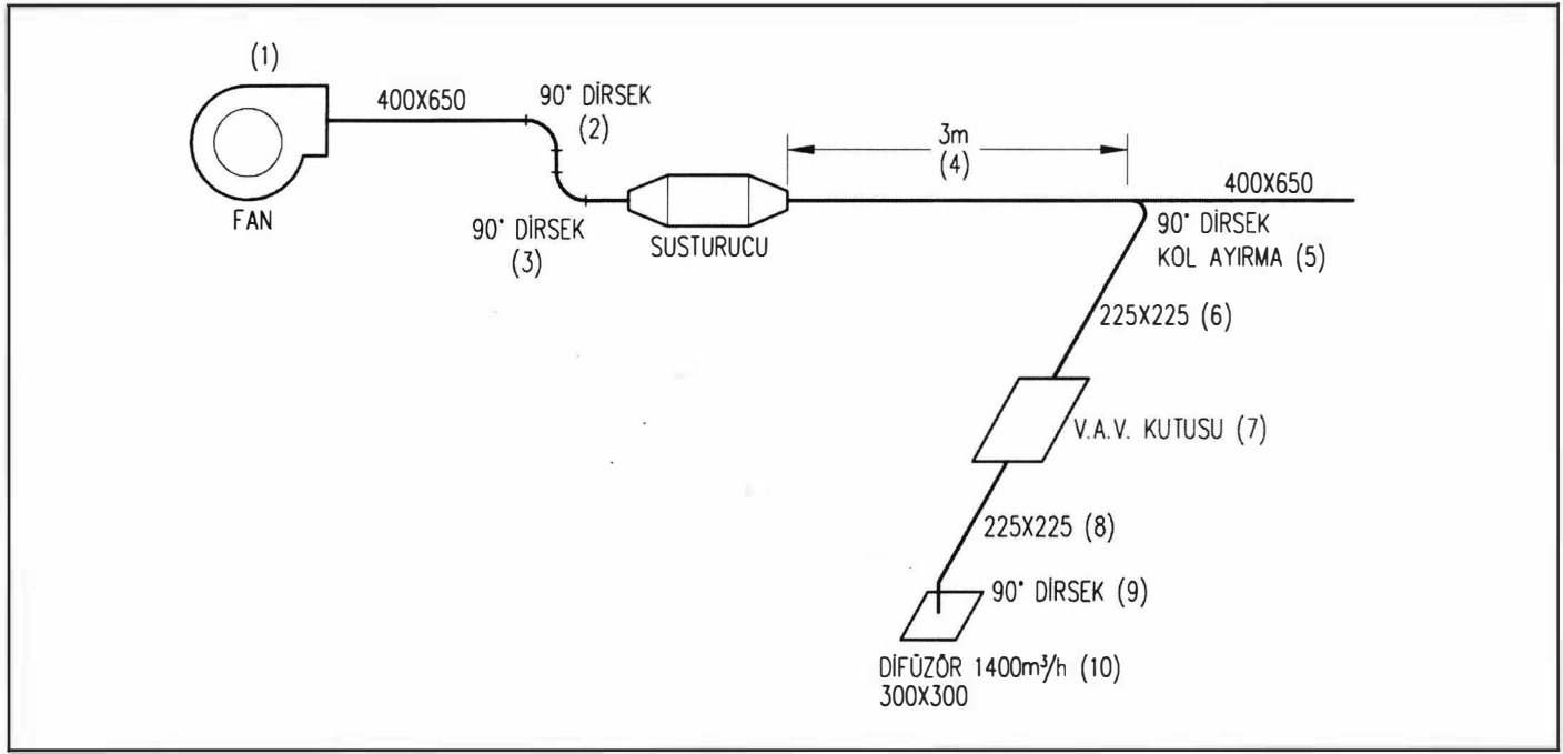
Şekil 2.29. SİSTEM ŞEMASI
