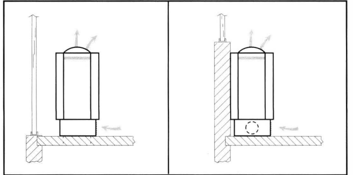
Şekil 17.70. KASETLİ DÖŞEME TİPİ (%100 İÇ HAVA)
