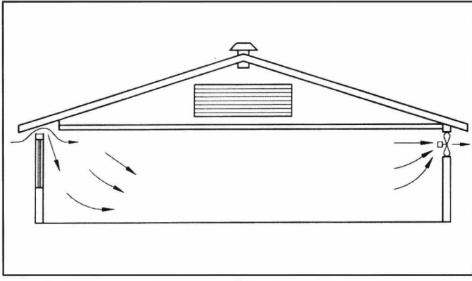
Şekil 14.61. EGZOZ ASPİRATÖRÜ VE YAN DUVARLARDAN GİRİŞ
