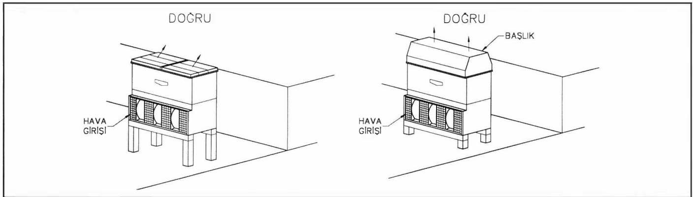
Şekil 17.26. KULE YÜKSELTİLİR VEYA BAŞLIK KULLANILIR
