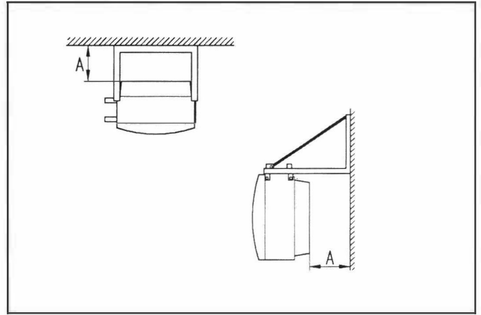
Şekil 17.97. İÇ HAVA İLE ÇALIŞAN APAREYLER İÇİN MONTAJ ARALIĞI
