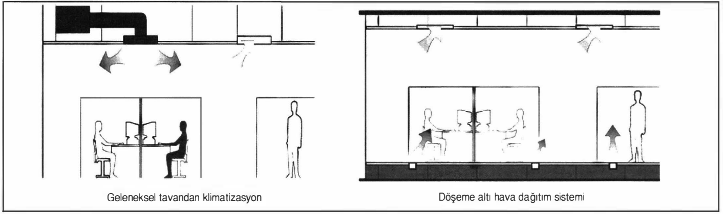
Şekil 11.35. GELENEKSEK TAVANDAN KLİMATİZASYON İLE DÖŞEMEDEN KLİMATİZASYON
