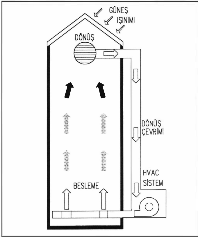
Şekil 14.21. GÜNEŞLİ VE SOĞUK KIŞ GÜNLERİNDE EKONOMİ ÇALIŞMASI
