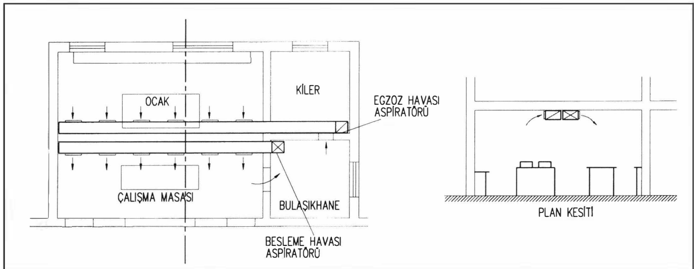
Şekil 14.51. BÜYÜK BİR RESTORANT MUTFAĞINDA BESLEME VE EGZOS HAVA KANALLARI
