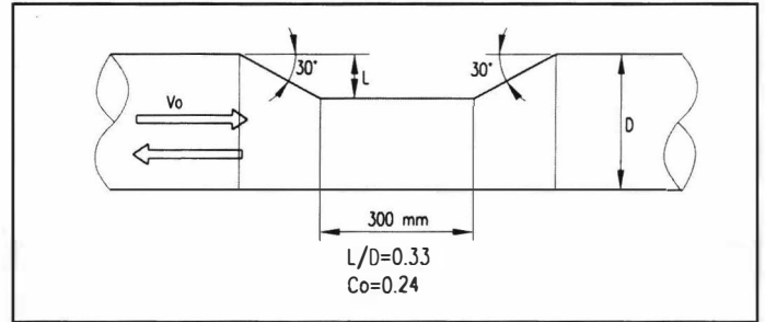
Şekil 21.12. KİRİŞ GEÇİŞİ
