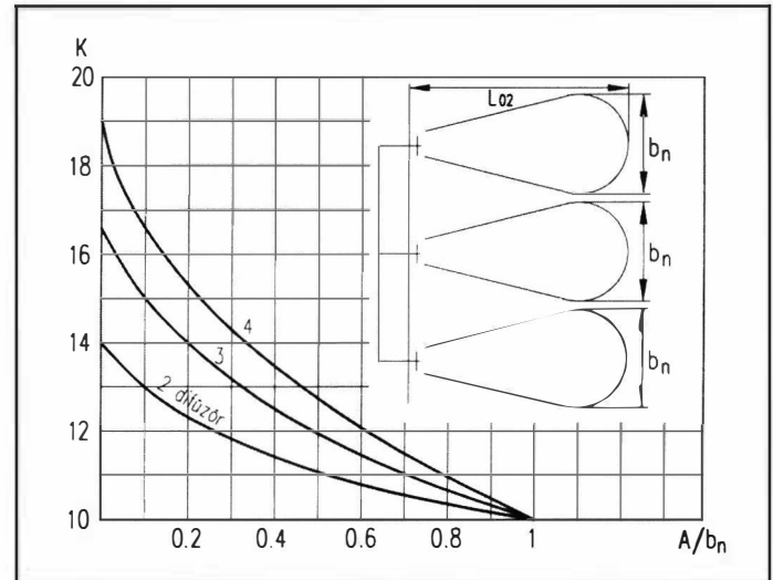
Şekil 4.6. K FAKTÖRÜ
