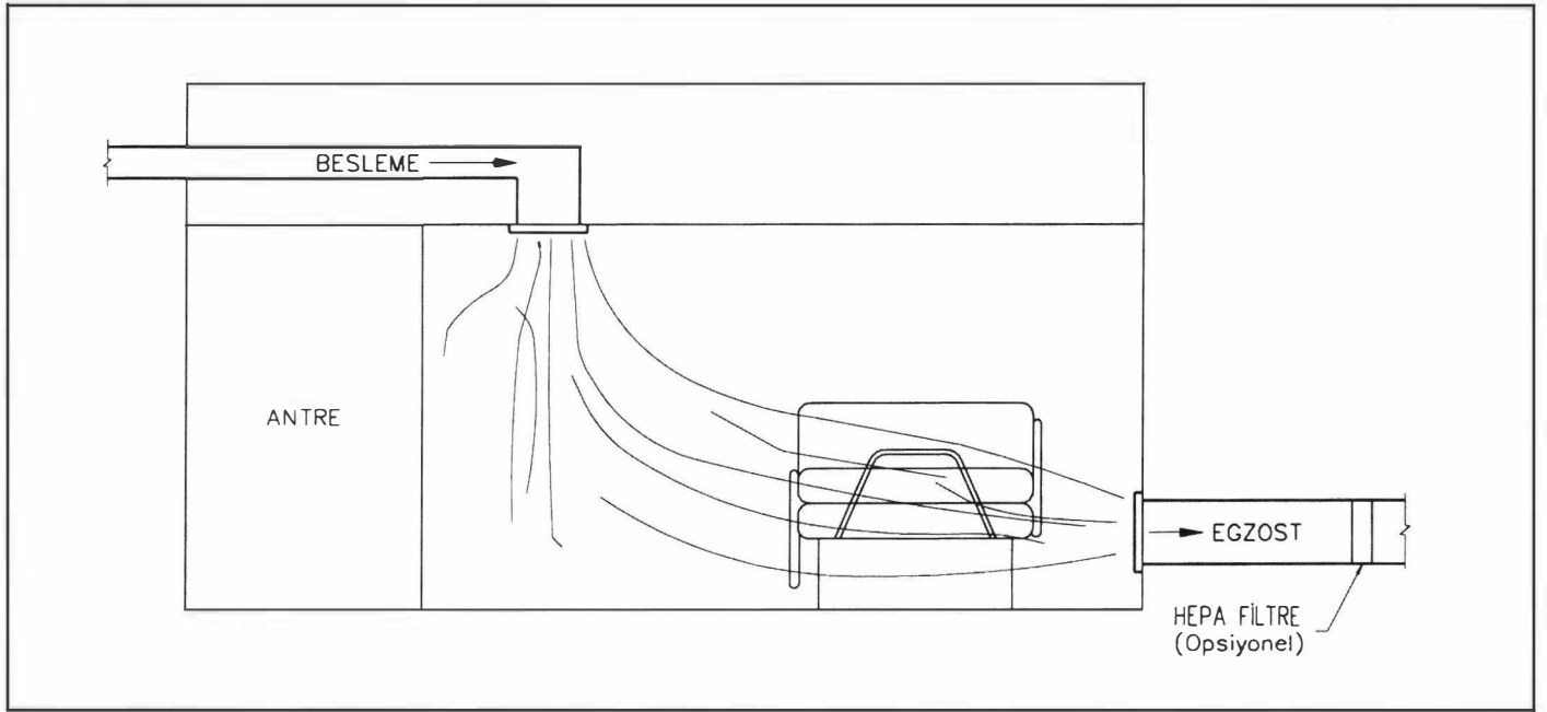
Şekil 16.11. DUVARDAN EGZOZLU KARANTİNA ODASI HAVA AKIŞI
