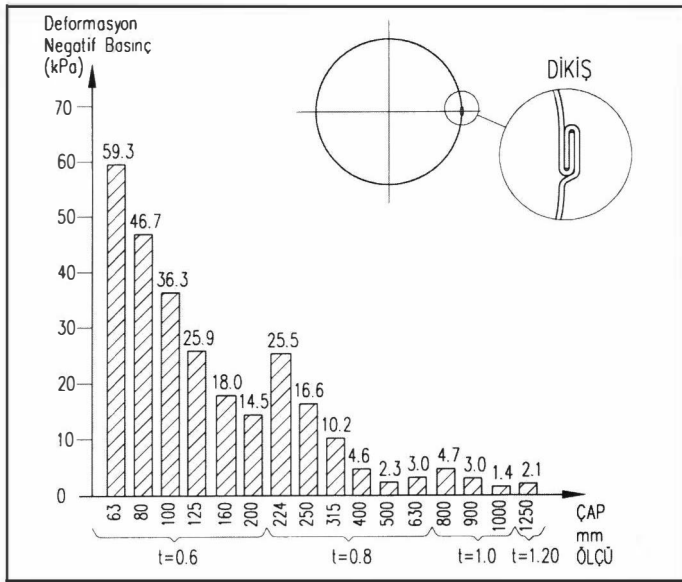
Şekil 1.67. YUVARLAK SİRAL KANAL NEGATİF BASINÇ DAYANIMI VE ET KALINLIĞI
