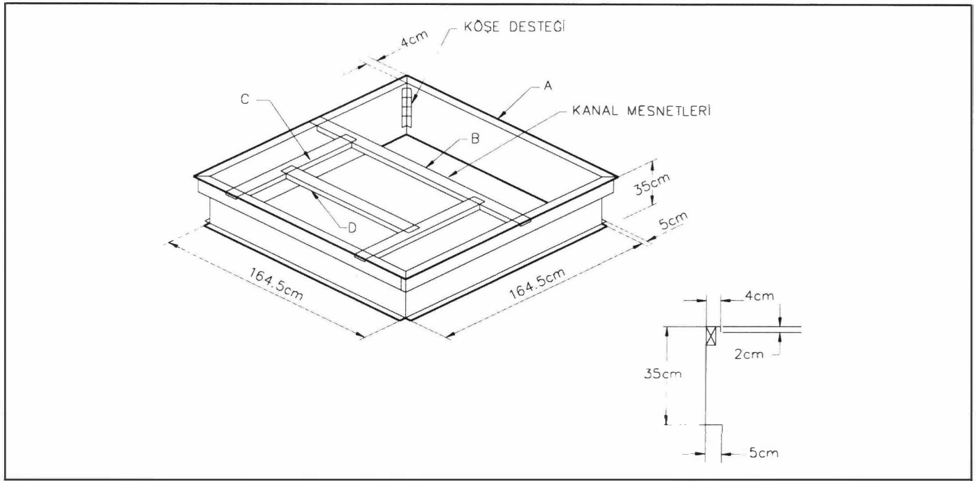
Şekil 12.68. ÇATI PLATFORMU
