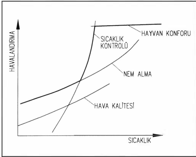
Şekil 14.60. OPTİMUM HAVALANDIRMA
