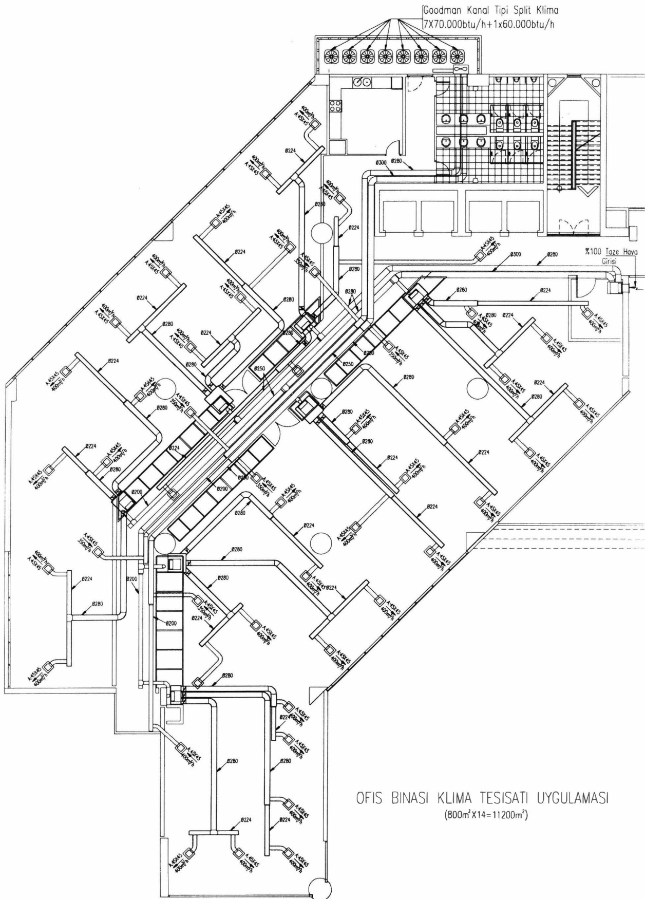
Şekil 11.34. ÇOK KATLI BİNA AMERİKAN SİSTEM KLİMA UYGULAMASI ÖRNEĞİ
