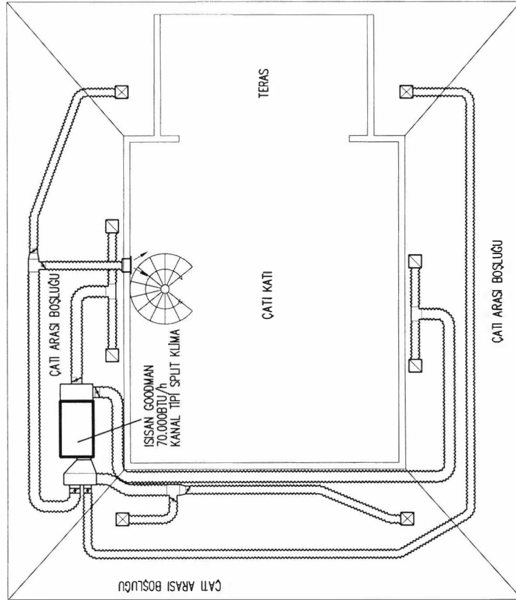
ÇATI KATI PLANI GOODMAN KANAL TİPİ SPLIT KLİMA UYGULAMASI
