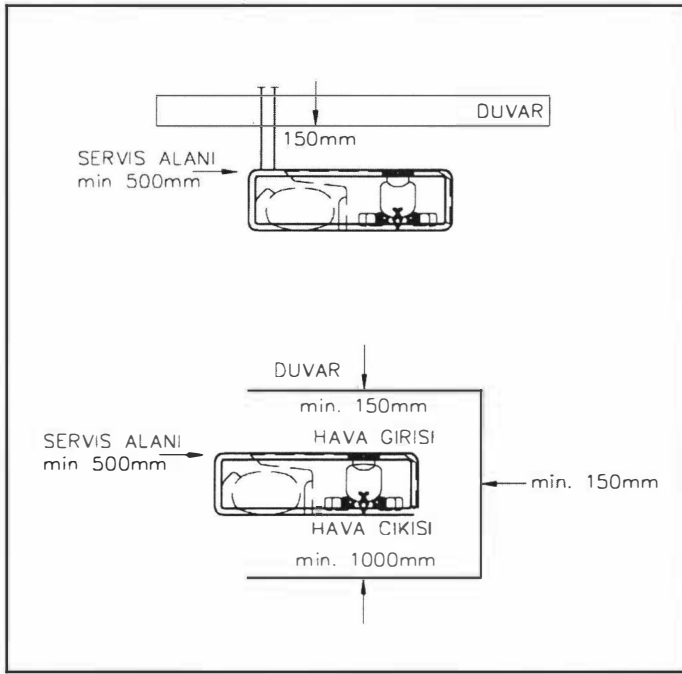
Şekil 12.3.A. ÜNİTE ETRAFINDA SERVİS ALANI OLMALIDIR
