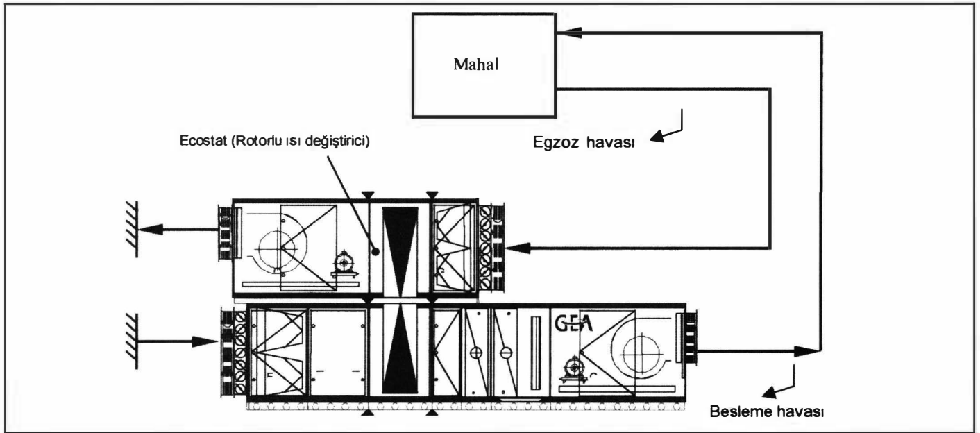
Şekil 17.55. ROTASYONLU ISI GERİ KAZANIM SİSTEMİ
