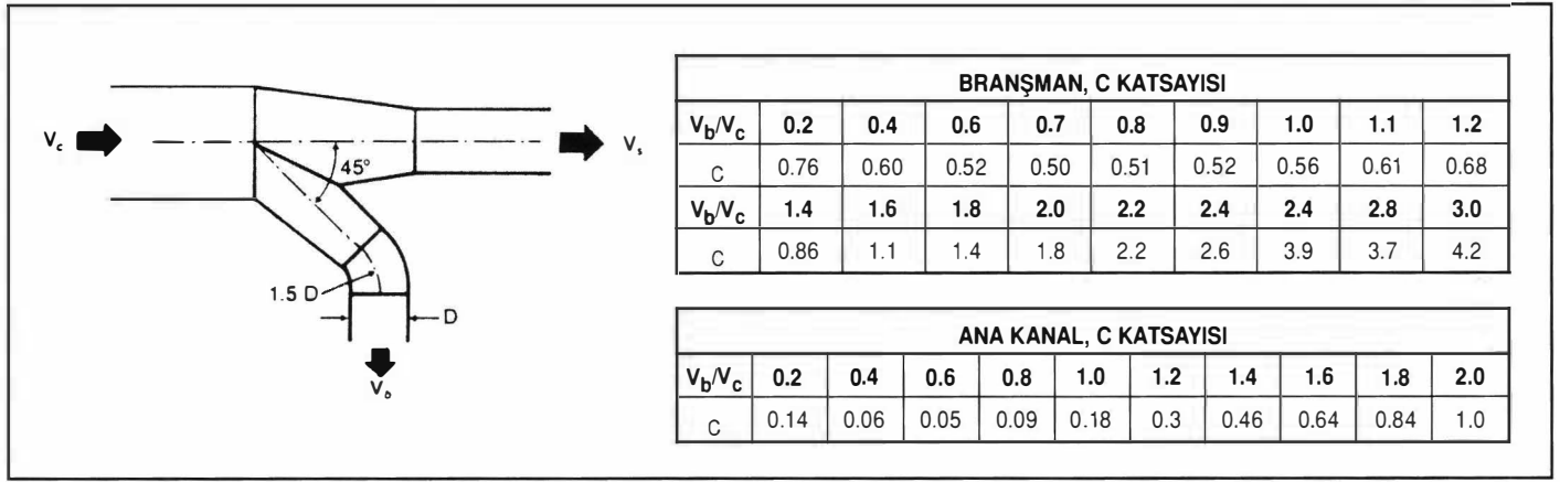
EK 2. Şekil 17. 45° W, KONİK ANA KANAL VE 45° DİRSEKLİ BRANŞMAN ANA KANALA 90°
