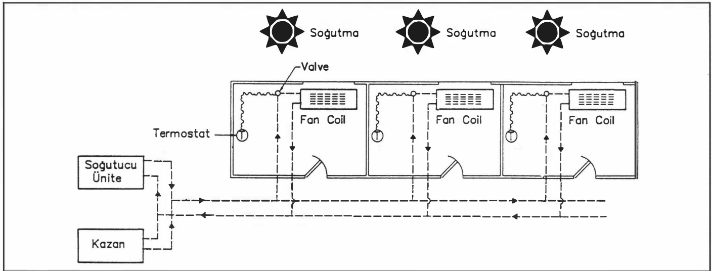
Şekil 11.10. 2 BORULU SİSTEM
