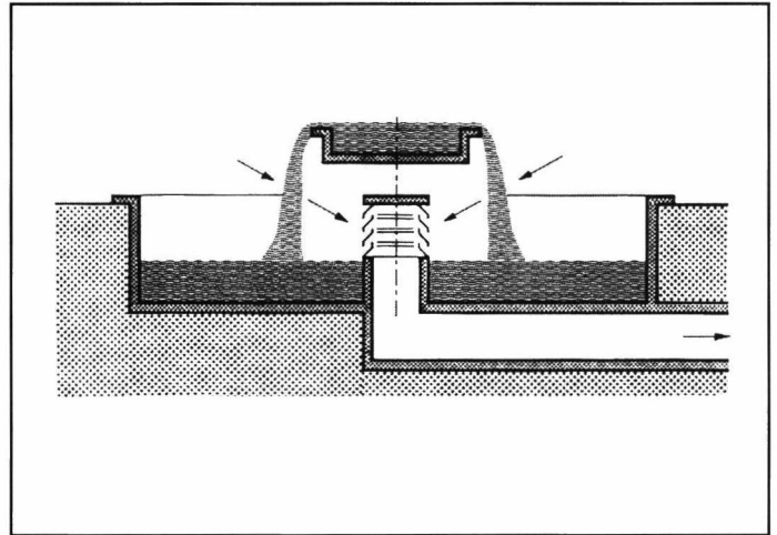
Şekil 4.28. HAVUZ ÜZERİNDEN HAVA EMİŞ ŞEMASI
