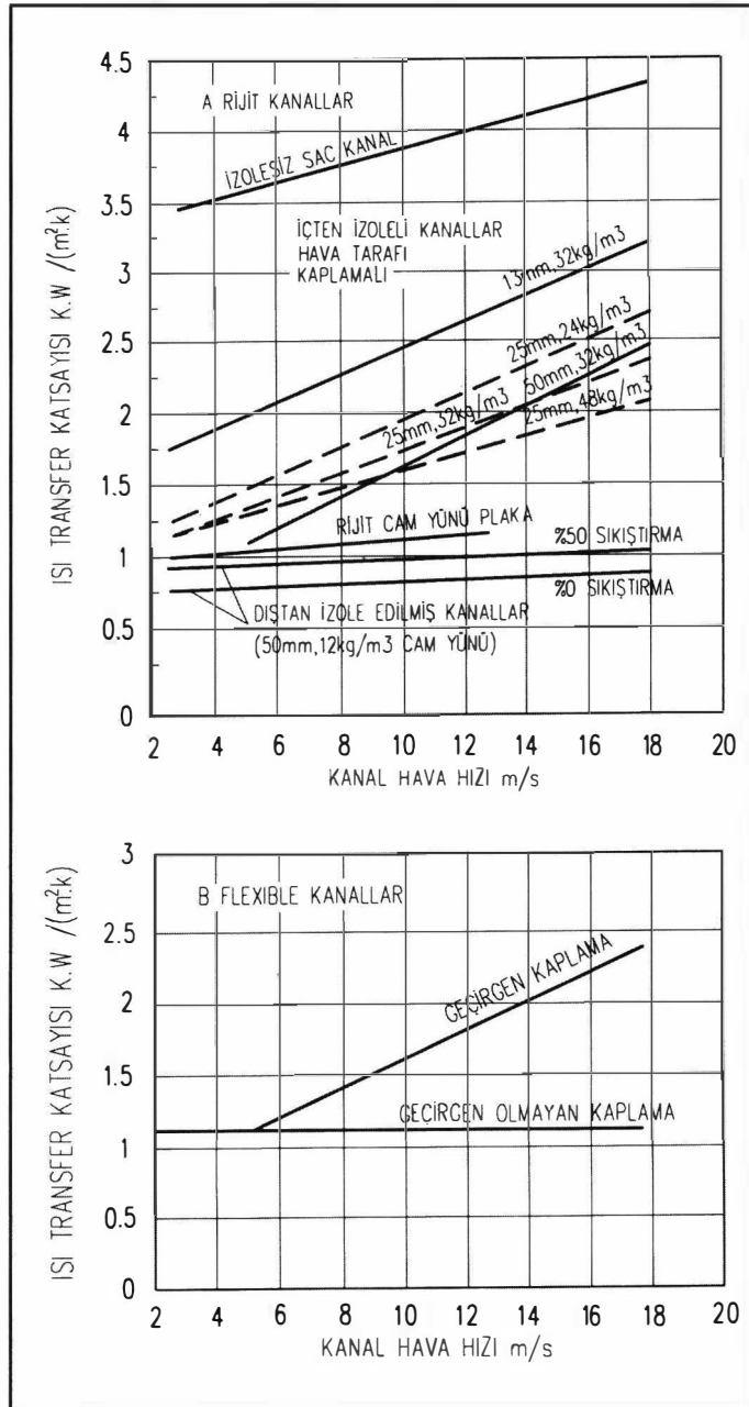
Şekil 1.16. KANAL ISI TRANSFER KATSAYILARI
