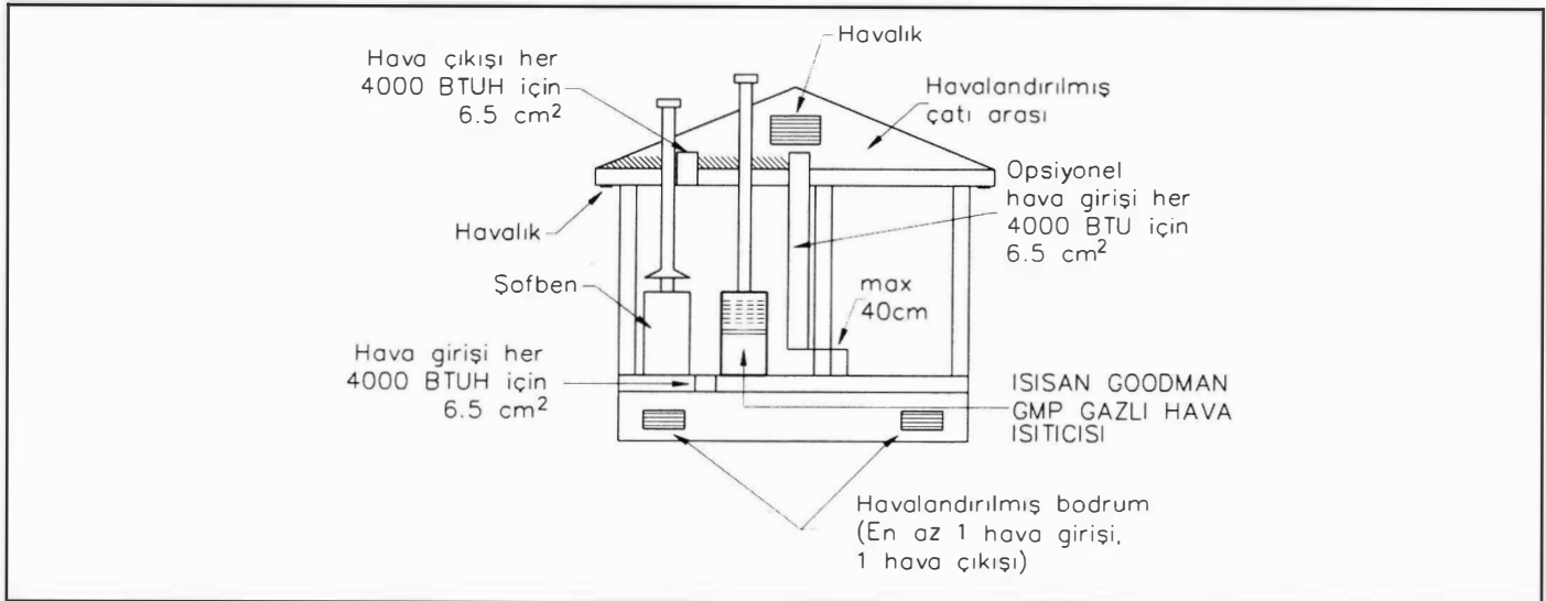
Şekil 12.52.A. ÇATI ARASINDAN VEYA BODRUMDAN HAVA ALIMI
