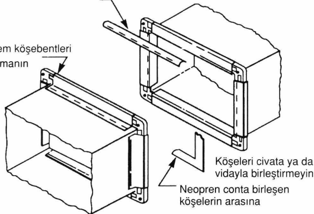
Şekil 6.19. UL TESTİNDEN GEÇMİŞ DAMPER BAĞLANTILARI
