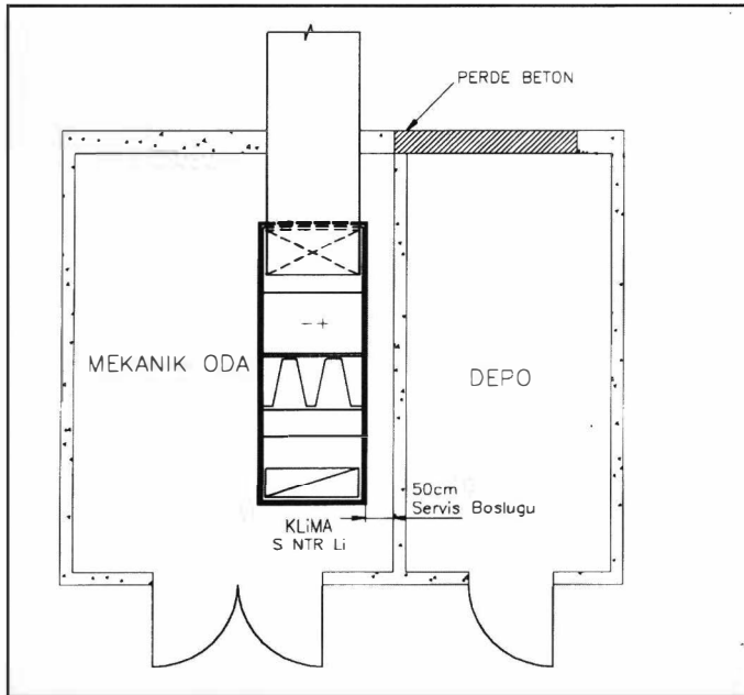
Şekil 1.63. ANA KANAL DÜZENLEMESİNDE DOĞRU ÇÖZÜM
