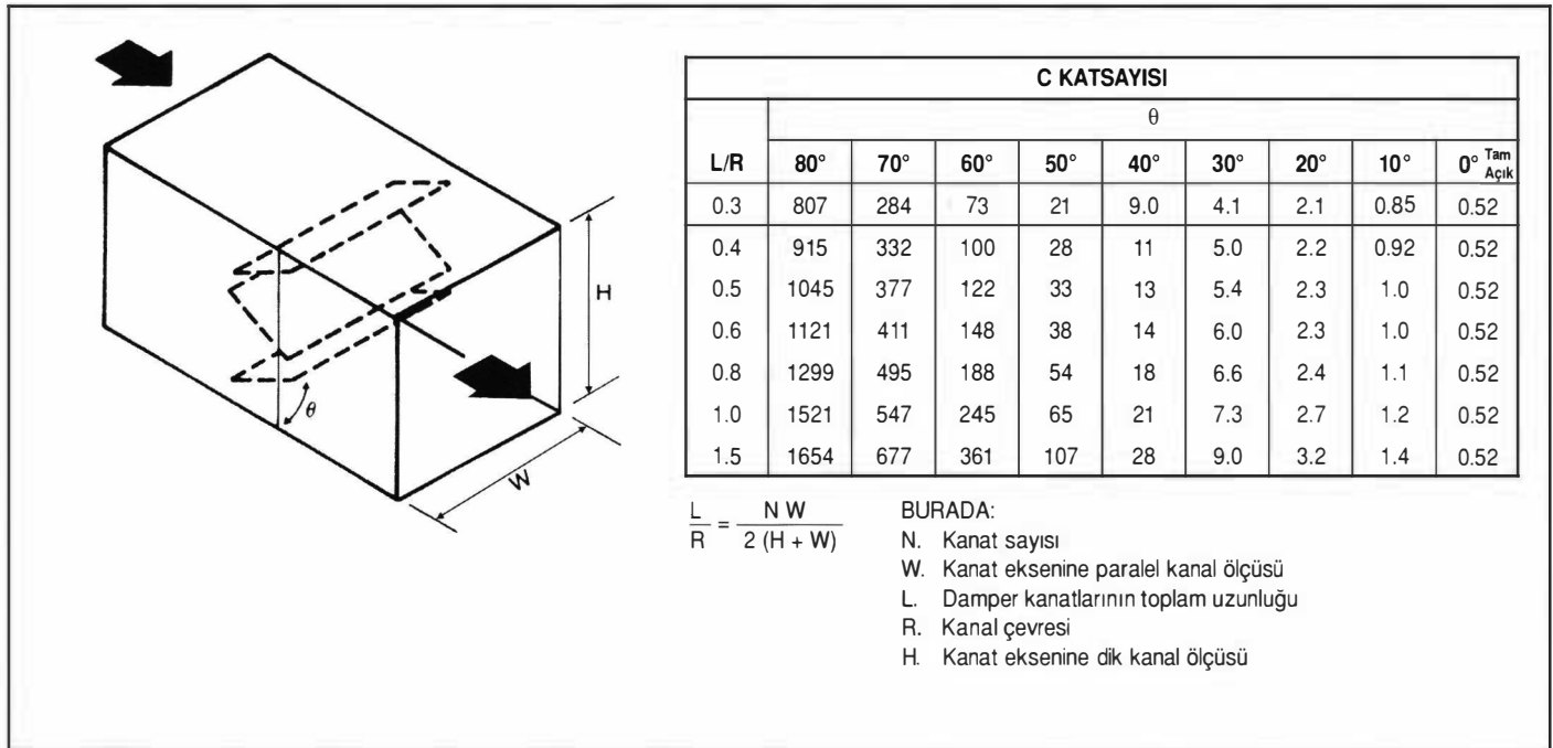
EK 2. Şekil 29. DAMPER, ÇOK KANATLI DİKDÖRTGEN
