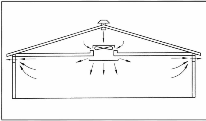
Şekil 14.63. BESLEME FANI VE YAN DUVARLARDAN EGZOZ
