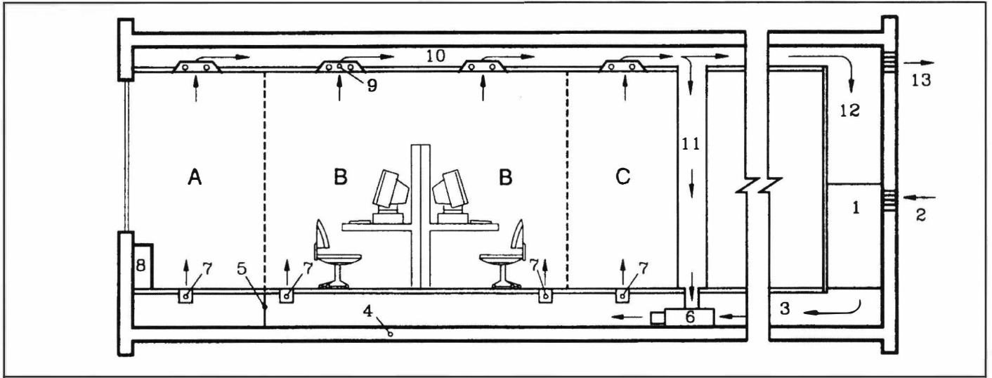
Şekil 11.37. DÖŞEMEDEN KLİMATİZASYON UYGULAMASI
