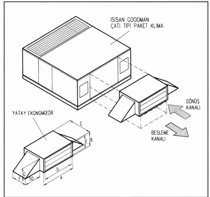
Şekil 12.73. YATAY EKONOMİZÖR
