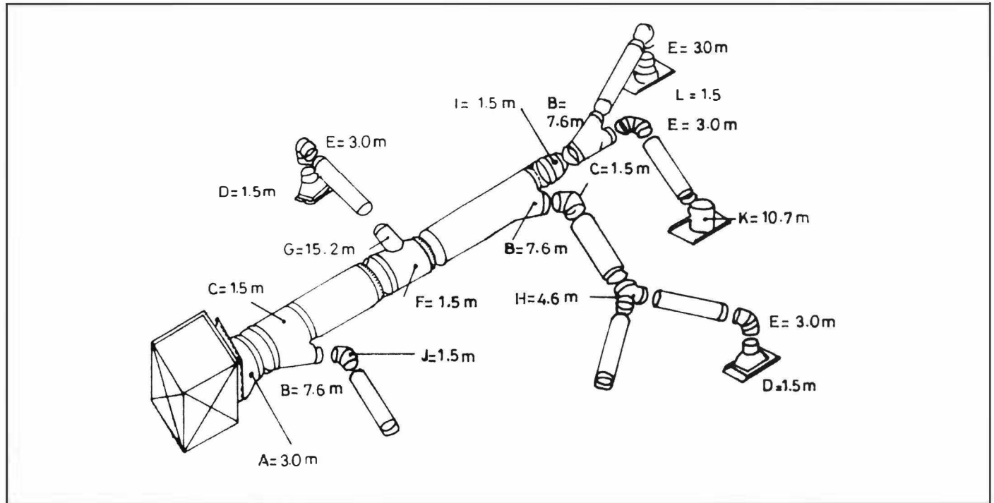
Şekil 12.36. EŞDEĞER UZUNLUKLAR
