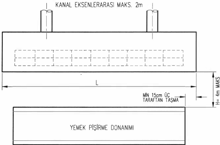
AÇIKTA DAVLUMBAZ
