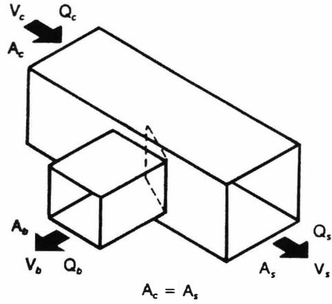
EK 2. Şekil 21. T PARÇA, DAMPERLİ BRANŞMAN VE ANA KANAL DİKDÖRTGEN
