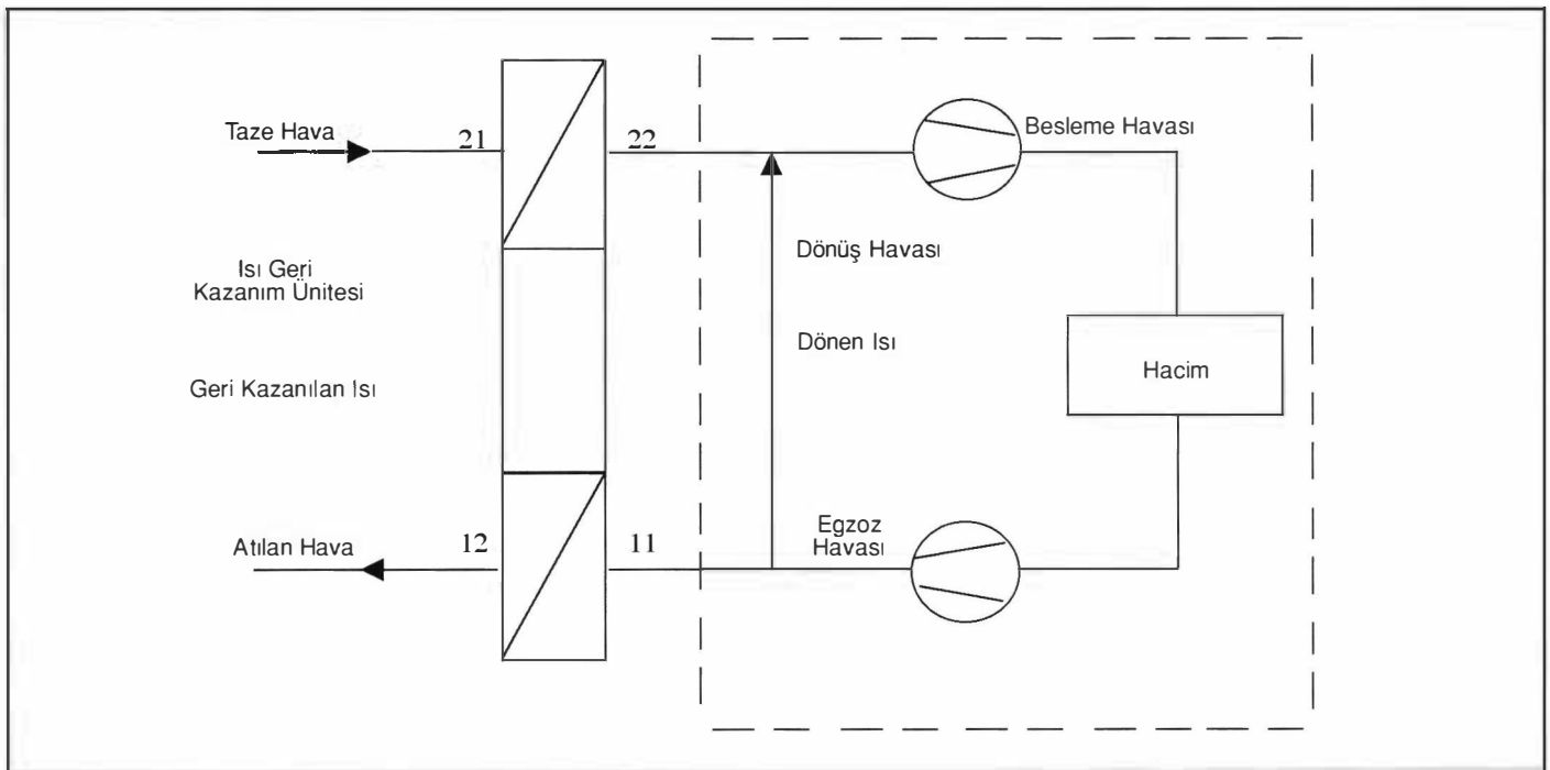
Şekil 17.51.A ISI GERİ KAZANMA SİSTEMİ ŞEMASI
