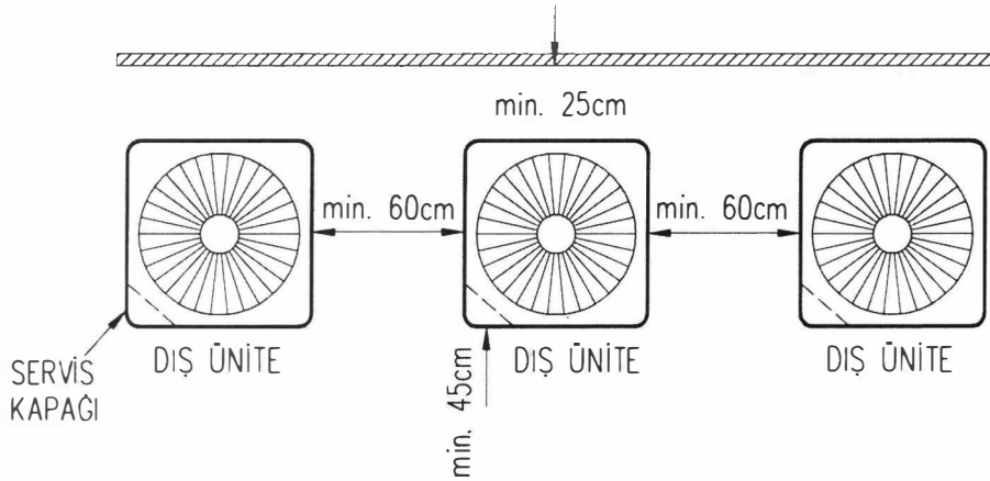
Şekil 12.10. ISISAN GOODMAN KANAL TİPİ SPLIT KLİMA DIŞ ÜNİTE YERLEŞİMİ (ÜSTTEN GÖRÜNÜŞÜ)
