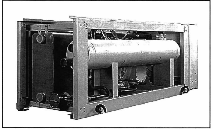
Şekil 17.2. SU SOĞUTMALI SU SOĞUTMA GRUBU
