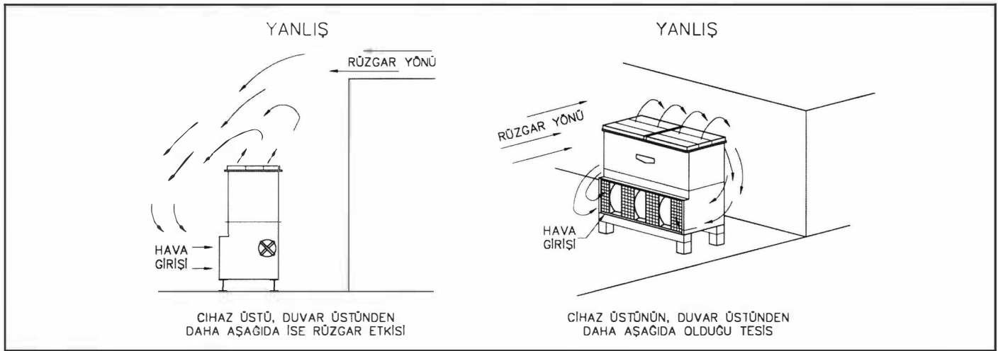
Şekil 17.25. KULE HAVA ÇIKIŞ SEVİYESİ DUVARIN ALTINDA OLMAMALIDIR
