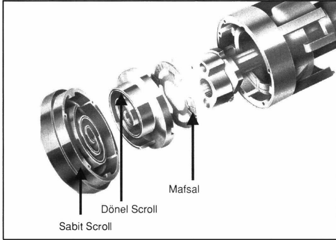
Şekil 17.9. SCROLL KOMPRESÖR BİLEŞENLERİ
