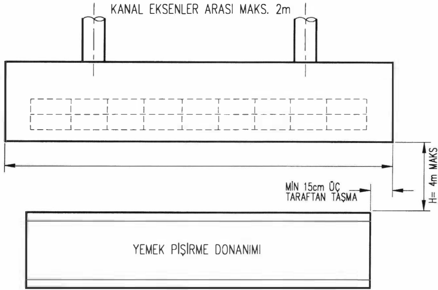
DUVARA DAYALI DAVLUMBAZ
