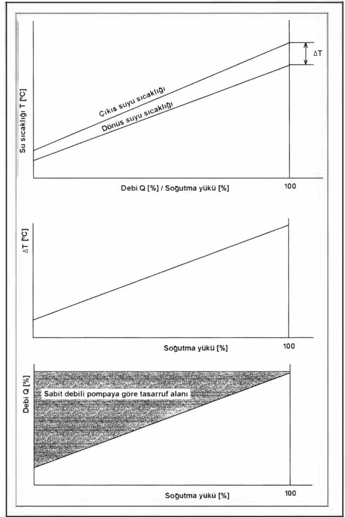
Şekil 17.115. SABİT OLMAK ÜZERE DEBİ \Delta T REGÜLYASYONU
