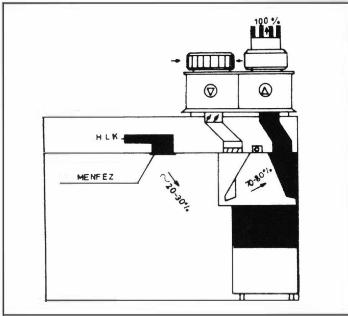
Şekil 14.58. ISI TASARRUFLU DAVLUMBAZ
