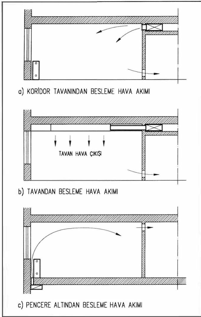
Şekil 14.26. DERSHANE HAVALANDIRMASI
