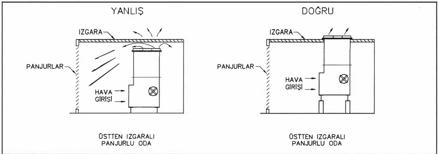
Şekil 17.32.C. IZGARA YAPIMI
