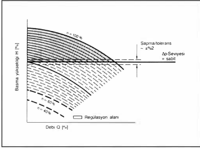
Şekil 17.114. DİFERANS BASINCI SABİT DÜZENLEME
