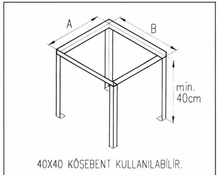
Şekil 12.14. İÇ ÜNİTE KAİDESİ
