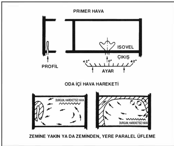
Şekil 4.15. GRUP C-ÇIKIŞLARI, HAVA HAREKETİ KARAKTERİSTİKLERİ
