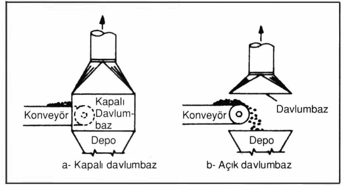
Şekil 7.10. AÇIK VE KAPALI DAVLUMBAZ
