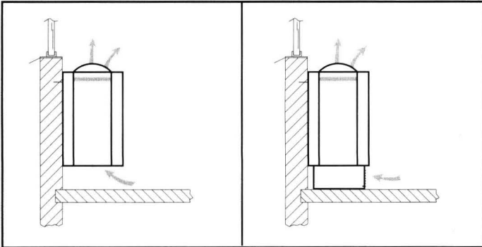
Şekil 17.69. KASETLİ DÖŞEME TİPİ (%100 İÇ HAVA) (ISITMA-SOĞUTMA)
