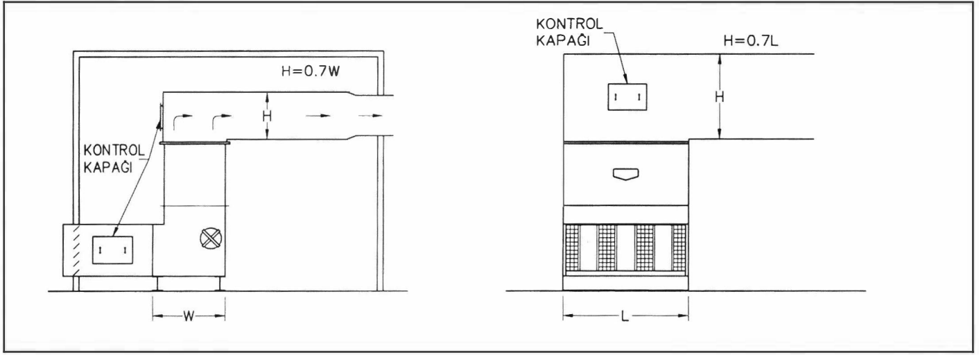
Şekil 17.32.D. KANAL KULLANIMI
