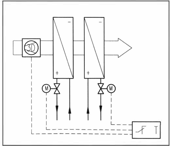
Şekil 11.17. DÖRT BORULU FAN COIL ISITMA VE SOĞUTMA KONTROL VANALI İKİ KONUMLU KONTROL
