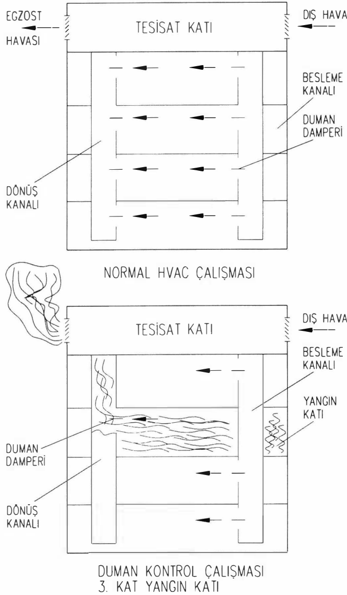
Şekil 6.7. MERKEZİ KLİMANIN DÜMEN TAHLİYESİNDE KULLANILMASI
