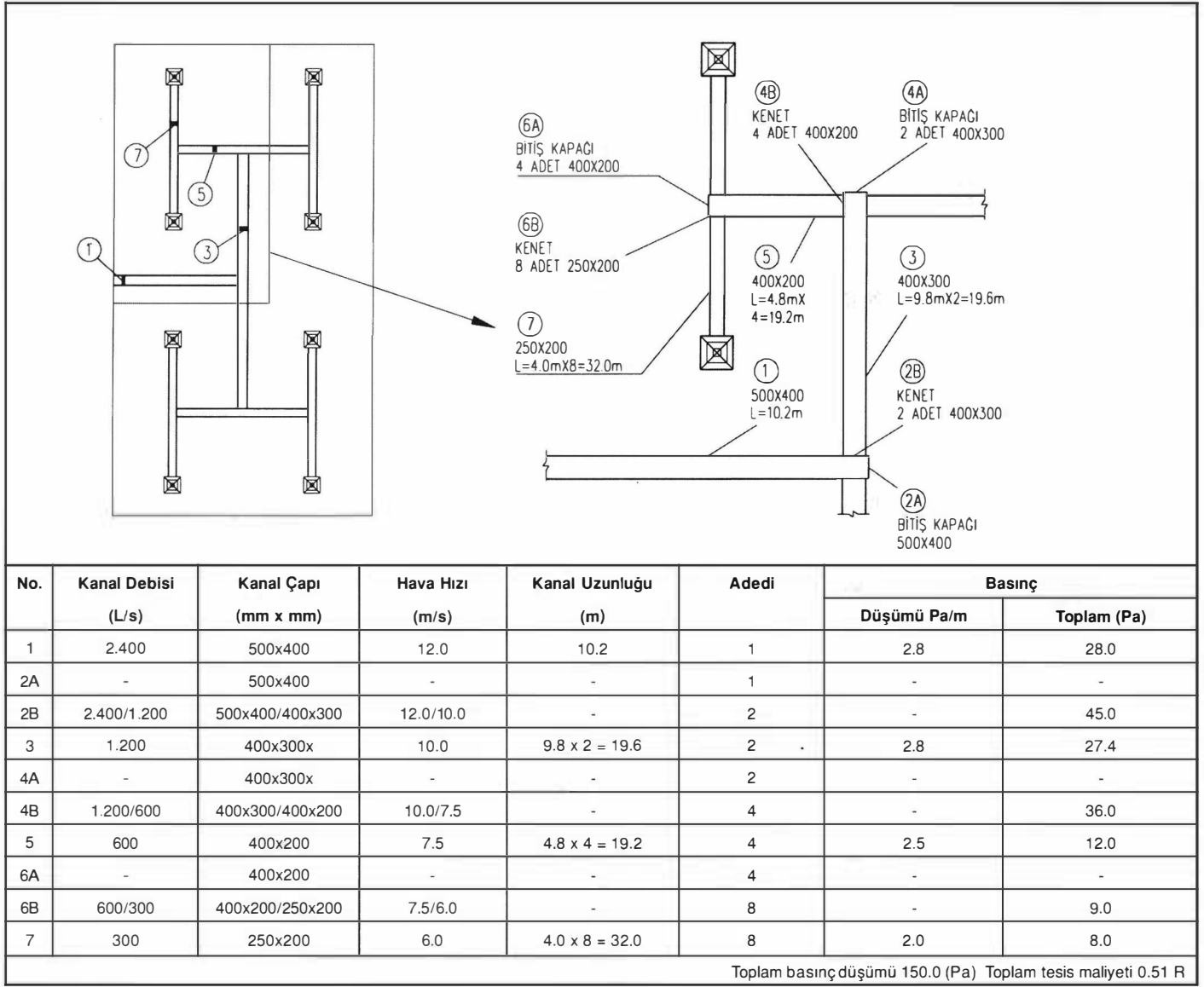
Şekil 1.79. DİKDÖRTGEN KANAL TESİSATI
