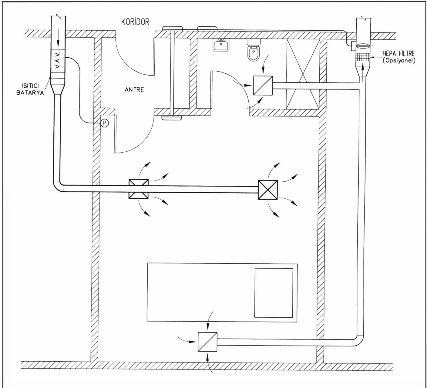
Şekil 16.13. İZOLASYON ODASI VAV BESLEME VE EGZOZLU KLİMA SİSTEMİ BASINÇ KONTROLU
