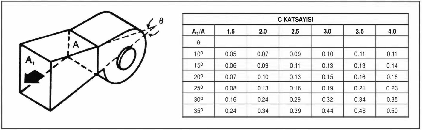
EK 2. Şekil 7. FANA GÖRE SİMETRİK, KENARLAR DÜZ GEÇİŞ PARÇASI
