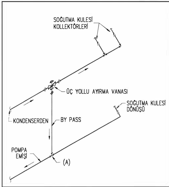
Şekil 17.20. KULE HATTI AYIRMA VANASI YERLEŞİMİ
