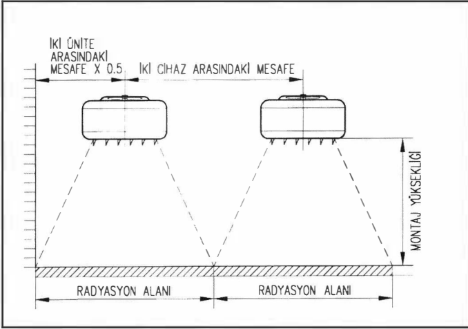
Şekil 17.91. TAVAN TİPİ APAREYLERİN RADYASYON ALANI
