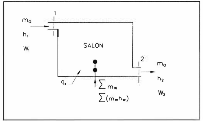
Şekil 10.21. BİR SALONDAKİ ISI VE NEM KAZANCININ NEMLİ HAVA İLE ALINMASINA AİT ŞEMA
