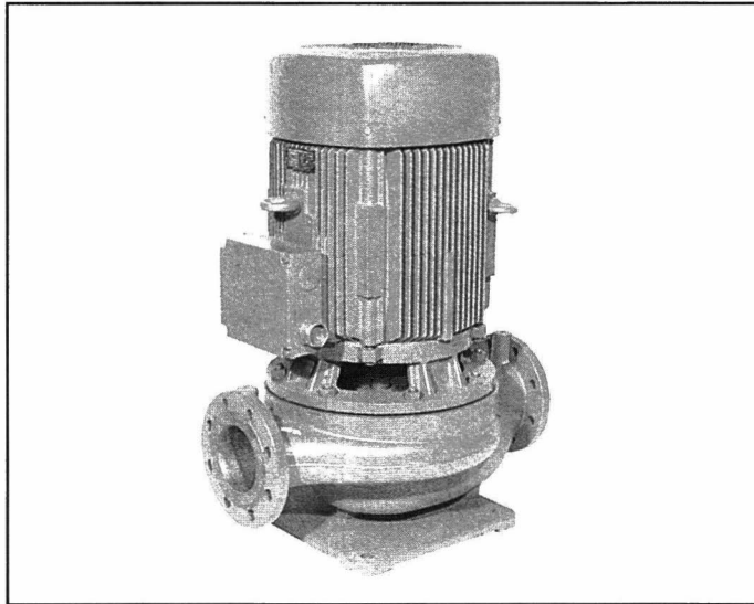
Şekil 17.103. BETON KAİDEYE BAĞLANABİLEN IN-LINE POMPA
