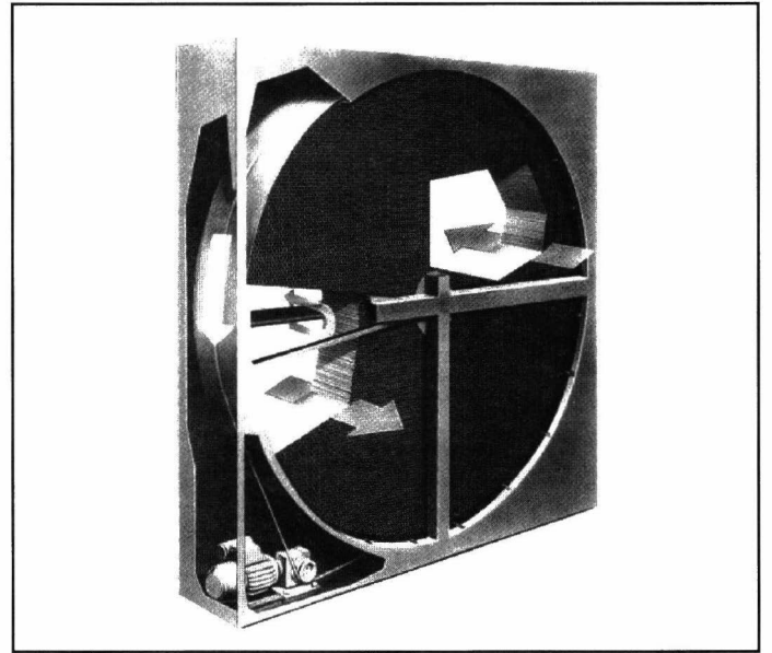
Şekil 17.51.C. ROTASYONLU ISI DEĞİŞTİRİCİ
