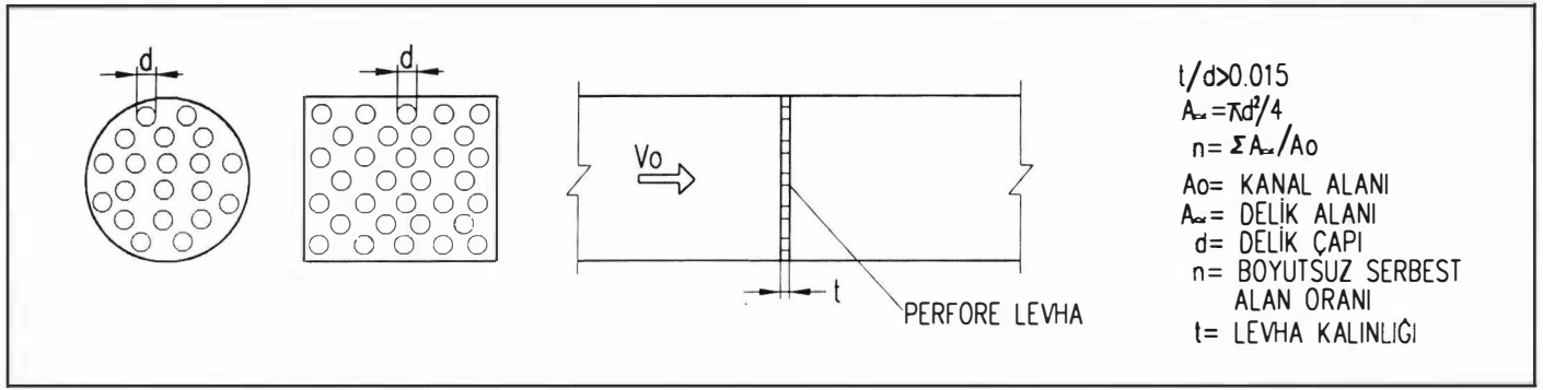
Şekil 21.13. DİRENÇ İÇİN PERFORE SAÇ KULLANIMI
