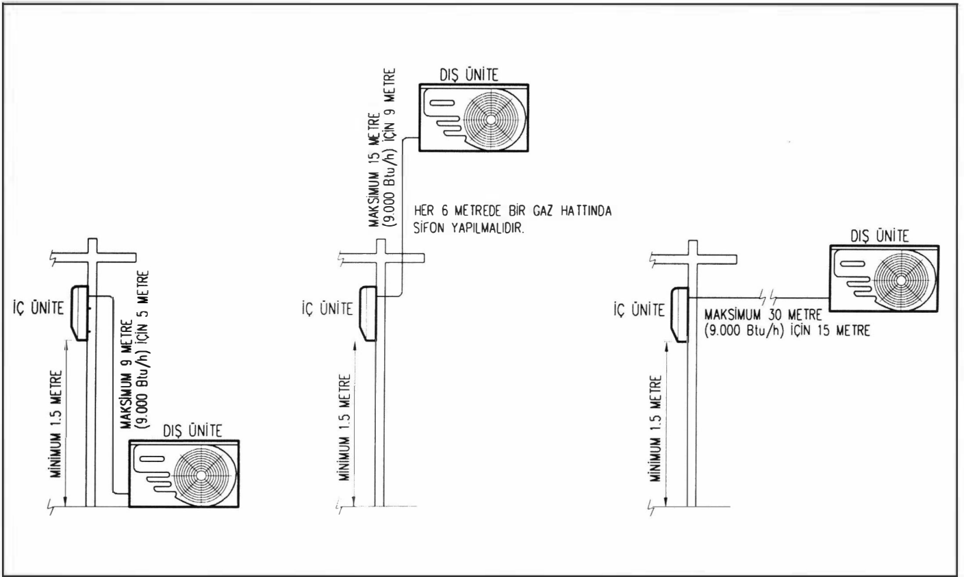
Şekil 12.84. ISISAN GOODMAN DUVAR TİPİ SPLIT CİHAZLARDA MAKSİMUM BAKIR BORU VE KOT FARKI ÖLÇÜLERİ
