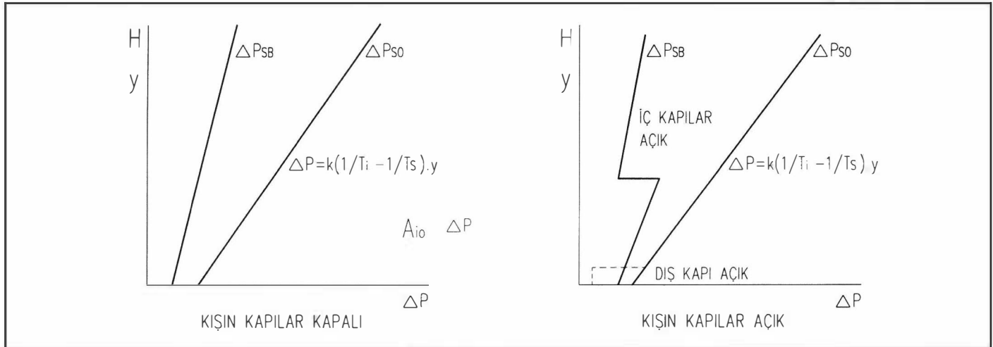
Şekil 6.16. Kışın bütün kapılar kapalı ve dış kapı açıkken basınç farkları
