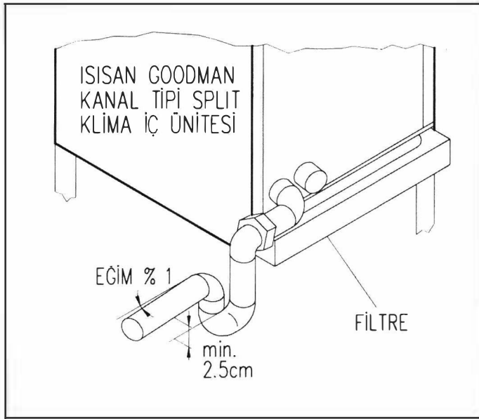
Şekil 12.11. DRENAJ BAĞLANTISI
