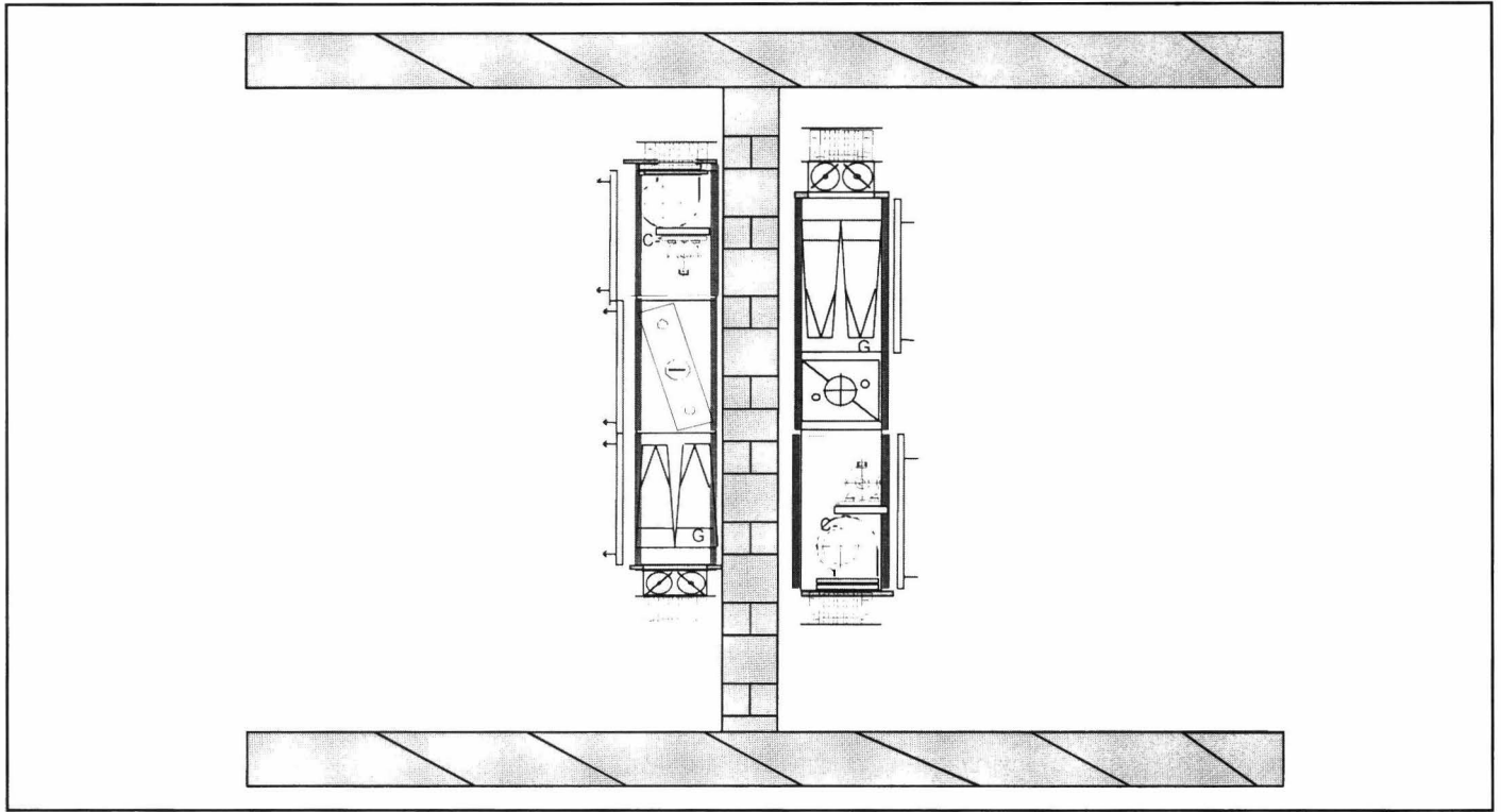
Şekil 17.48. ALÇAK TİP KLİMA SANTRALİ UYGULAMASI (GEA-AT PICCO ALÇAK TİP KLİMA SANTRALİ)
