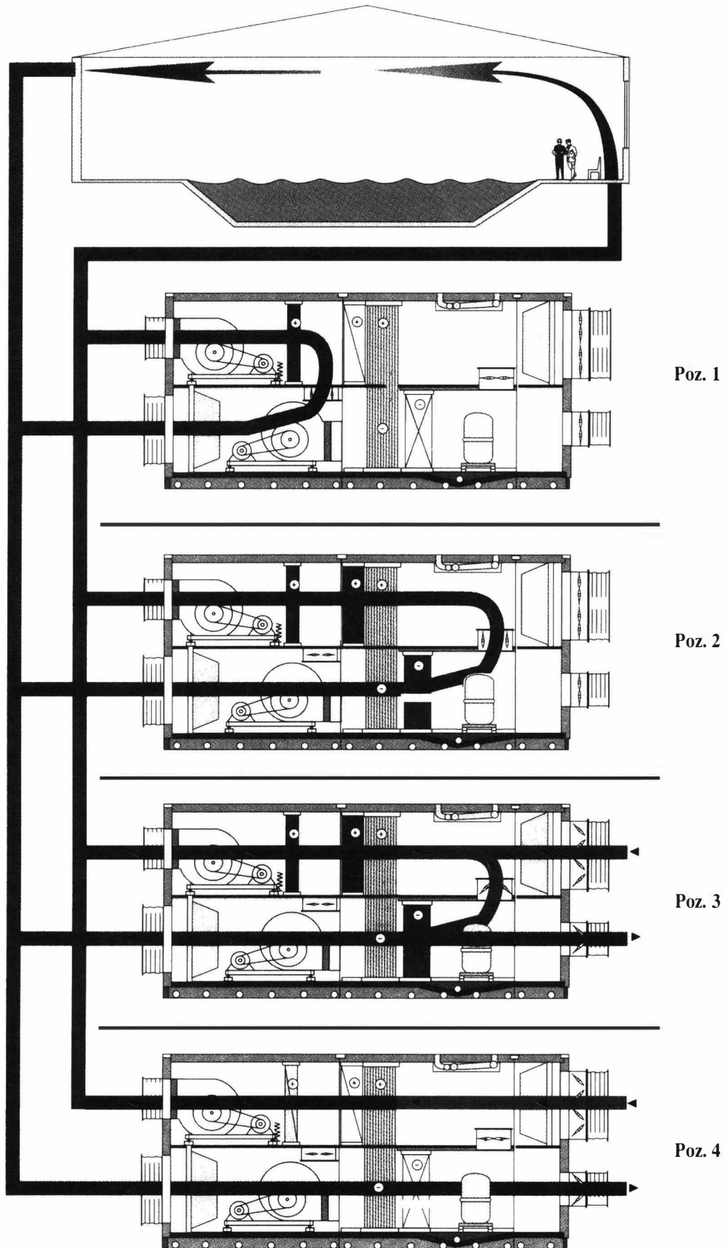
Şekil 14.42. HAVUZ KLİMA SANTRALİNİN ÇALIŞMA PRENSİBİ
