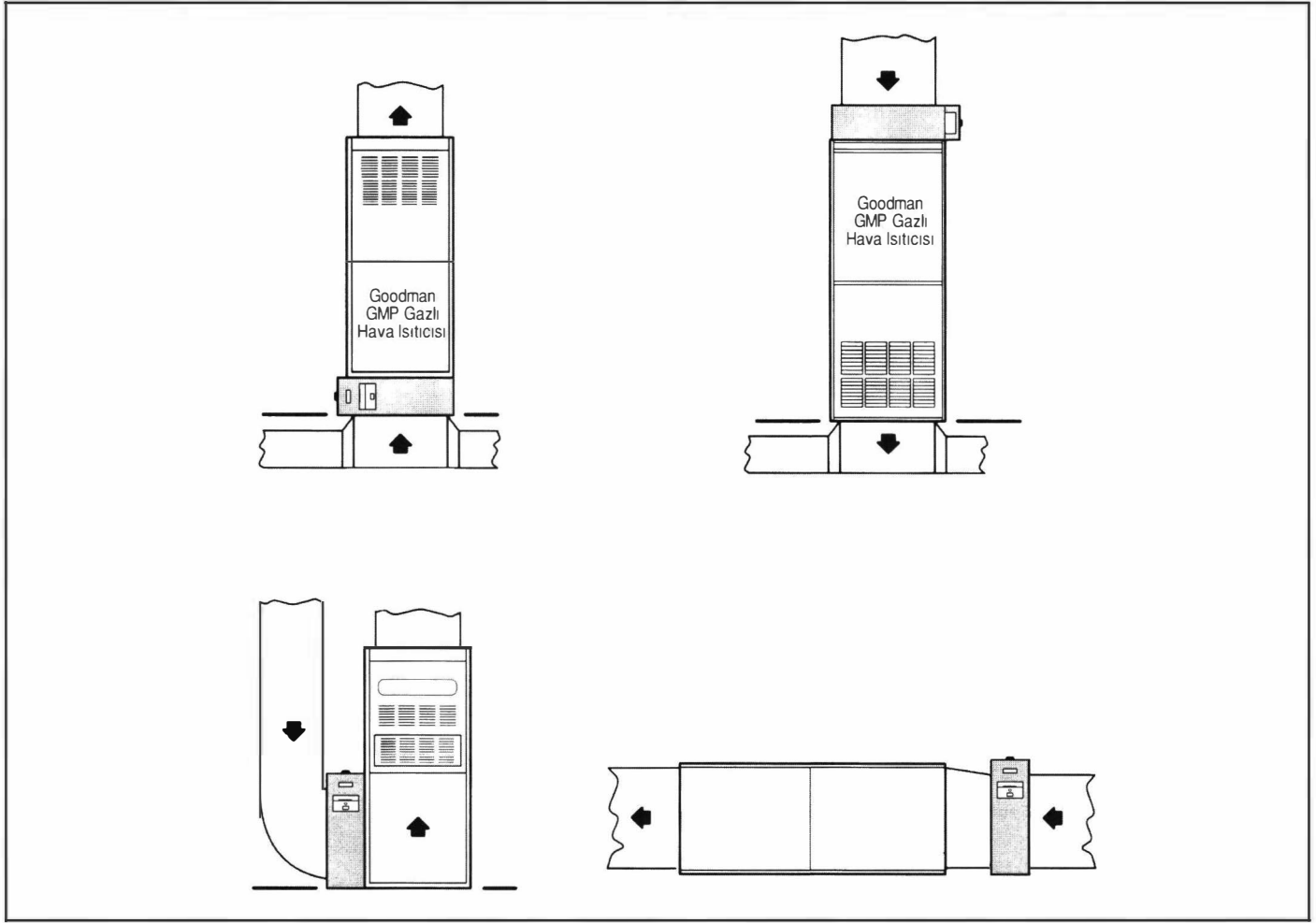
Şekil 12.80. MONTAJ ALTERNATİFLERİ
