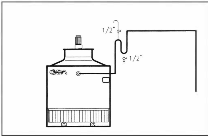
Şekil 21.20. KULE GİRİŞİNDE SİFON UYGULAMASI
