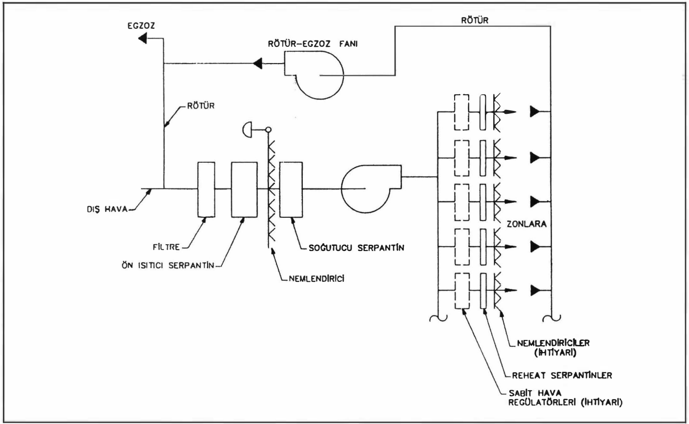
Şekil 11.2. REHEAT SİSTEMİ
