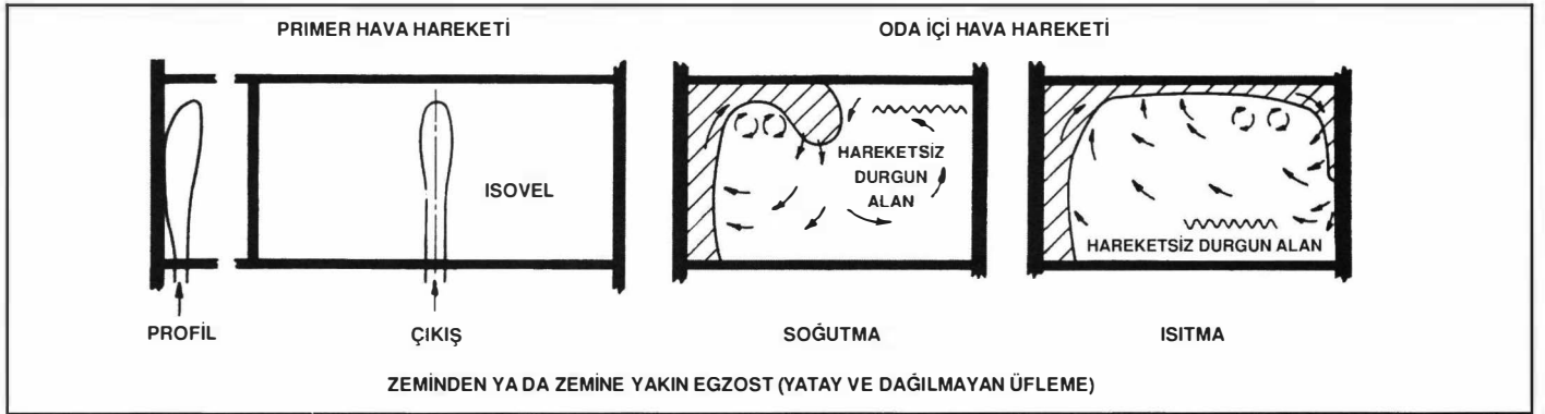
Şekil 4.14. GRUP B-ÇIKIŞLARI, HAVA HAREKETİ KARAKTERİSTİKLERİ
