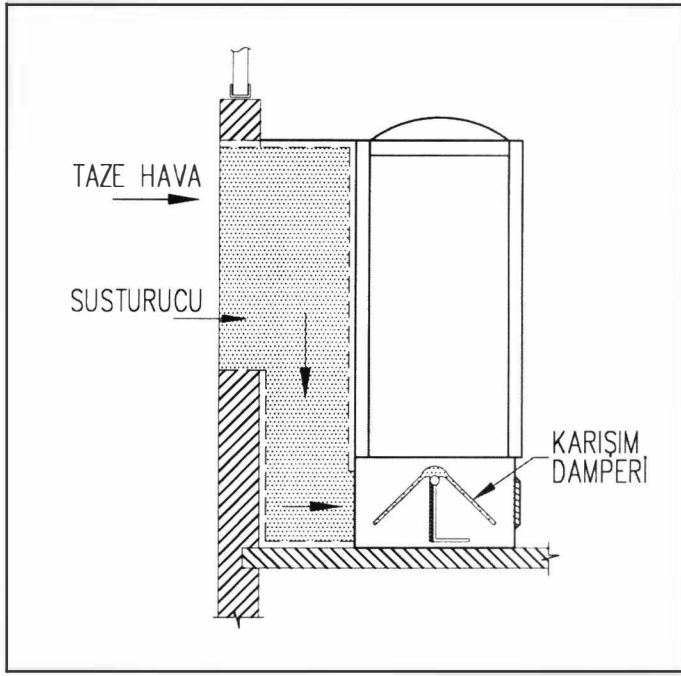
Şekil 17.80. KARIŞIM HAVALI DÖŞEME/TAVAN TİPLERİNDE SUSTURUCU KULLANILMASI
