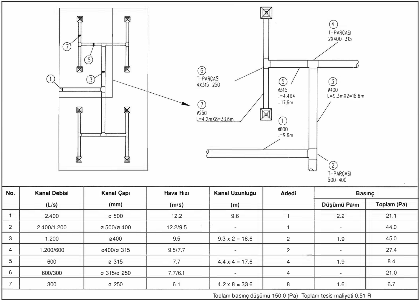
Şekil 1.80. YUVARLAK KANAL (VE FITTINGS) TESİSATI
