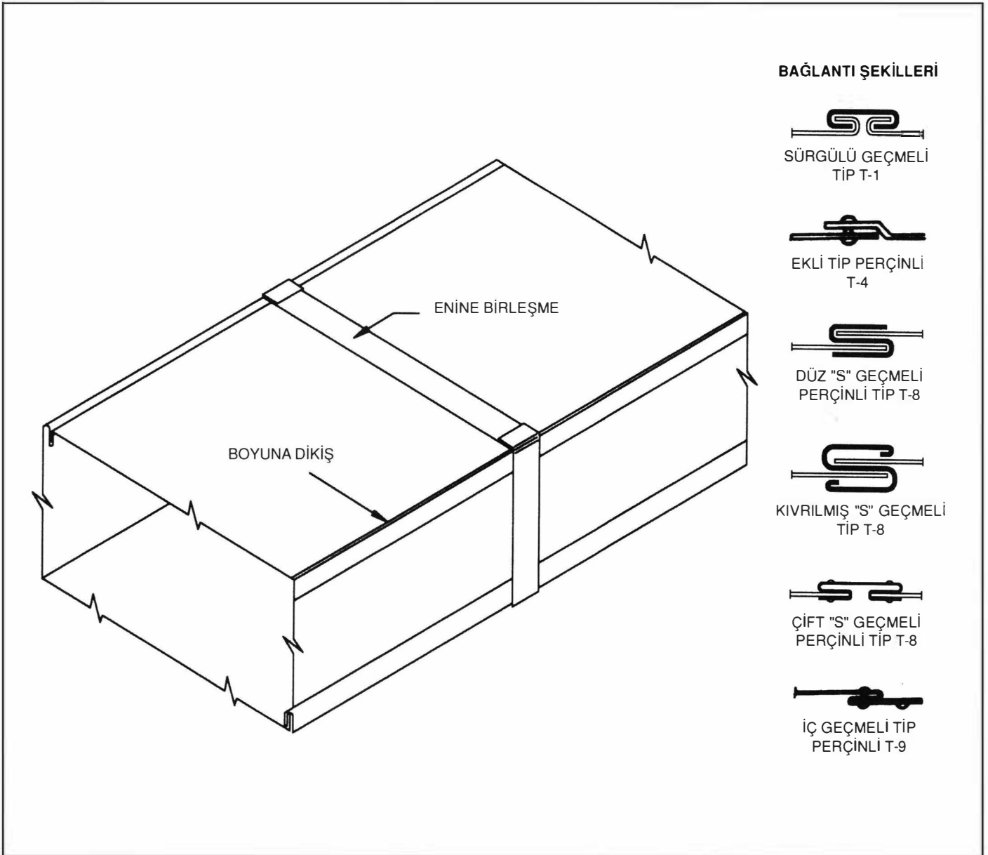
Şekil 3.2. TAKVİYESİZ KANAL
