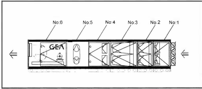
Şekil 17.61. DÖRT FİLTRASYON KADEMELİ MUTFAK ASPIRATÖRÜ
