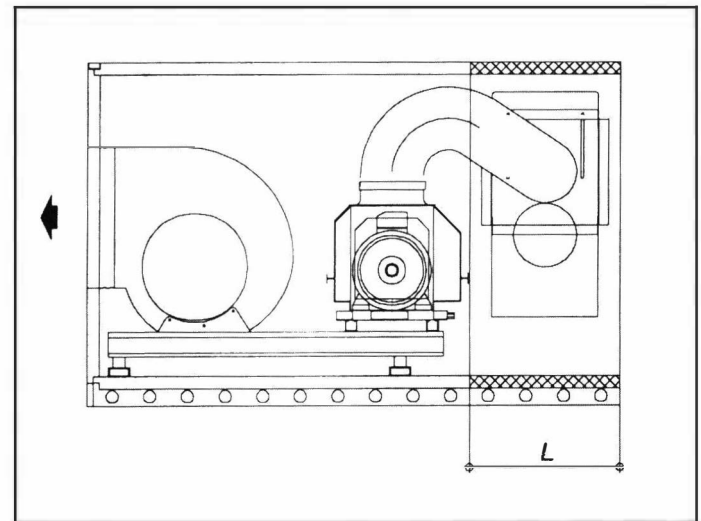
Şekil 17.62. HARİCİ HAVALANDIRMALI MOTOR
