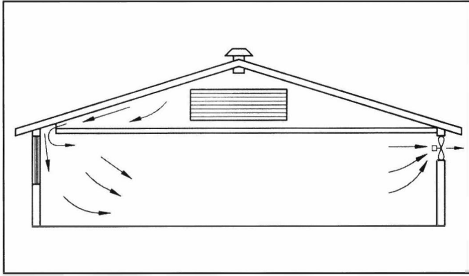
Şekil 14.62. EGZOZ ASPİRATÖRÜ VE ÇATI AÇIKLIKLARINDAN GİRİŞ
