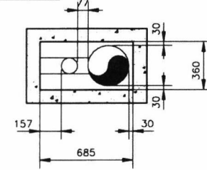
C-C Kesiti
