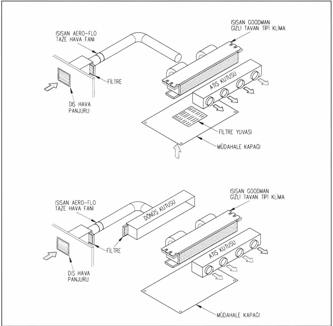
Şekil 12.32. ISISAN GİZLİ TAVAN TİPİ KLİMA TAZE HAVA BAĞLANTISI
