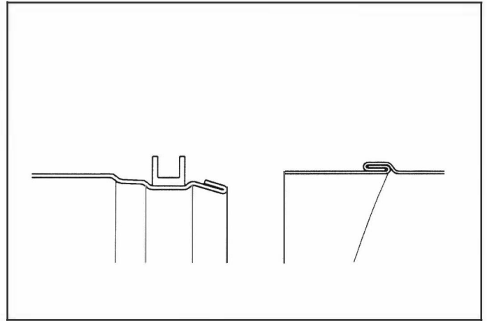
Şekil 1.84. SIZDIRMAZLIK CONTASI
