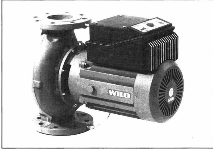
Şekil 17.109. FREKANS KONVERTER ENTEGRASYONLU KURU ROTORLU TEKİ TİP IN-LINE POMPA
