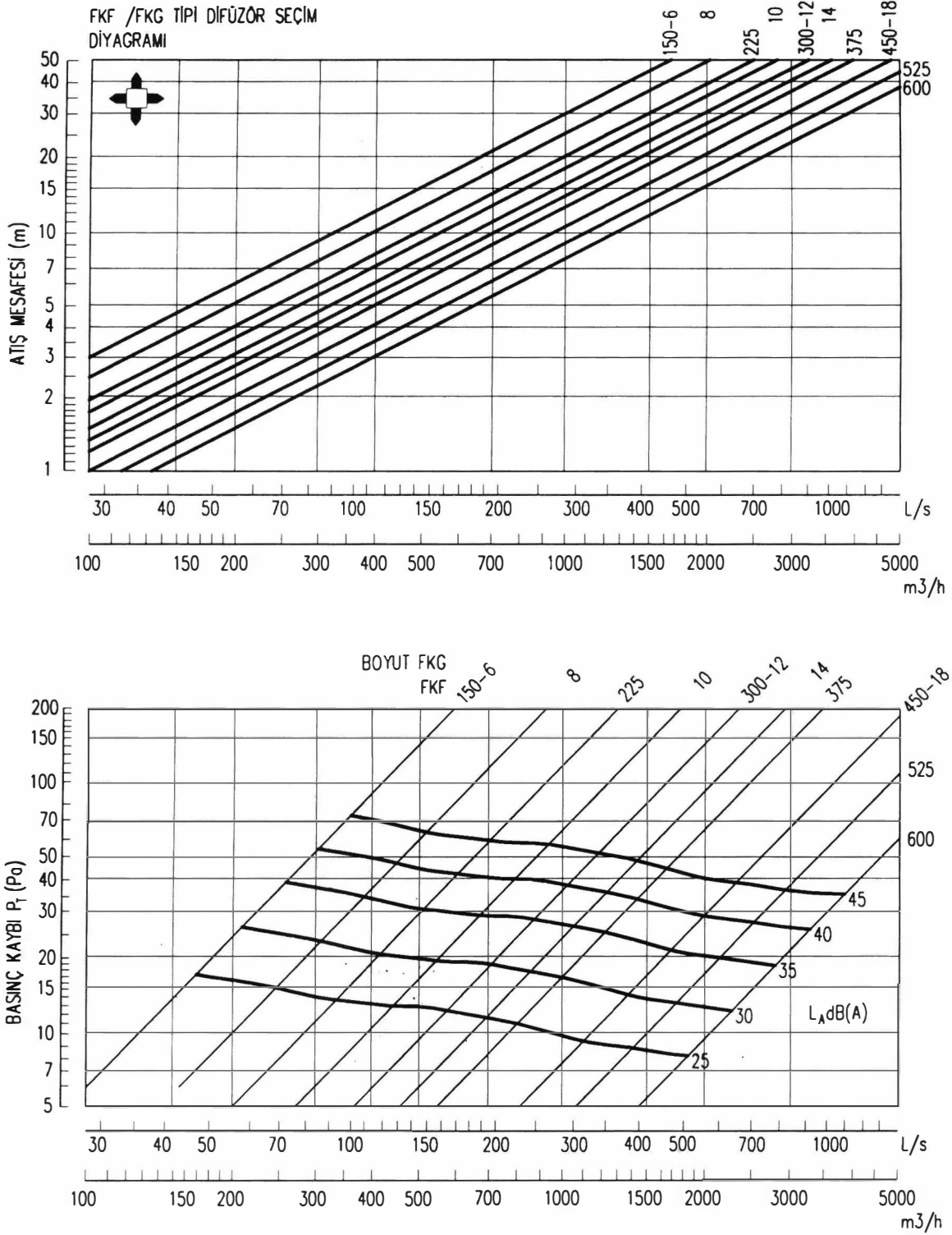
Şekil 4.26. FKF/FKG TİPİ DİFÜZÖR SEÇİM DİYAGRAMI
