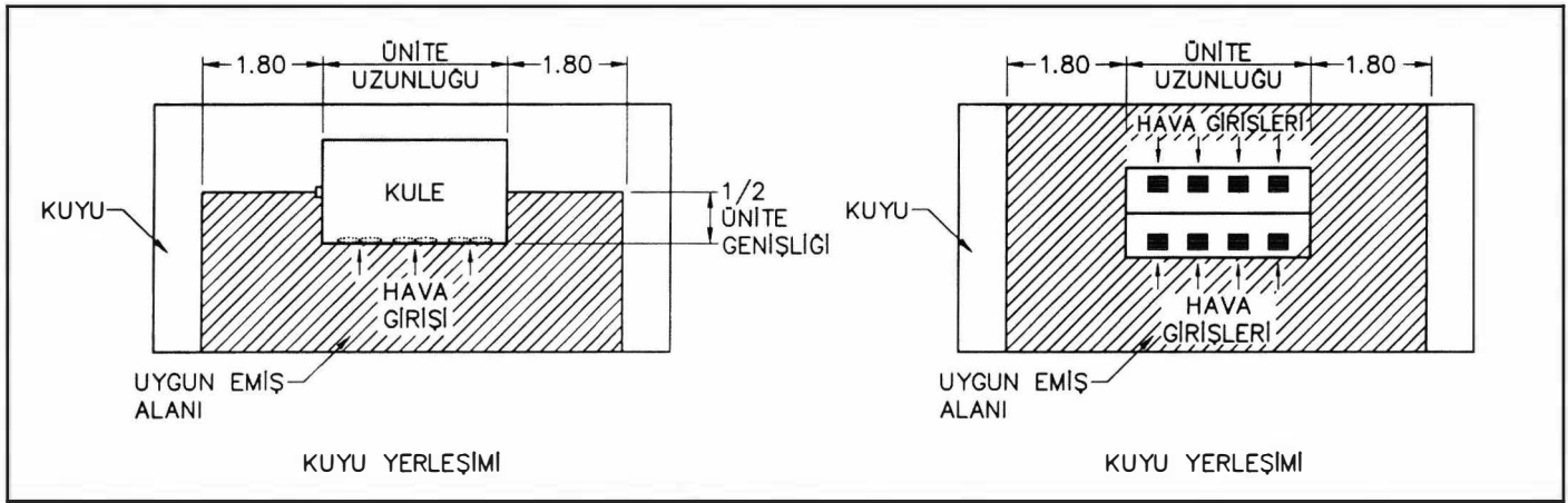
Şekil 17.31. KULE İÇİN GEREKLİ ALAN
