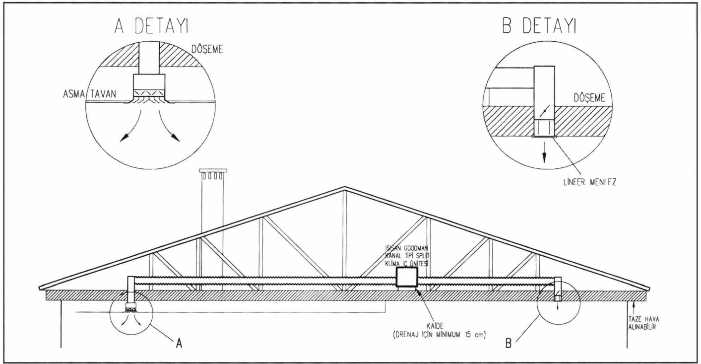
Şekil 14.2. ÇATI ARASI KANAL DAĞITIMI
