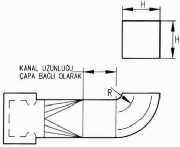
b) KARE KESİTLİ DİRSEK - 3 UZUN DÜZELTME KANATLI
