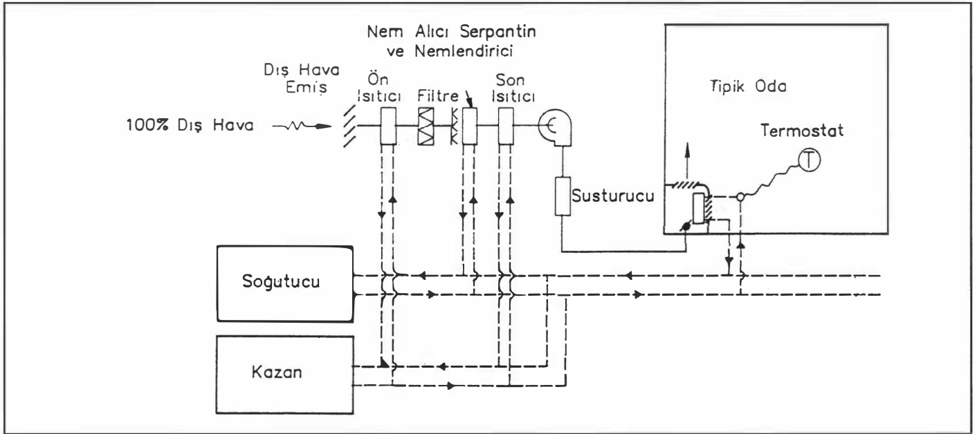
Şekil 11.19. ENDÜKSİYON
